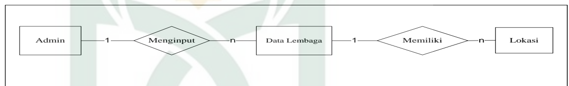
Gambar IV.8 ERD
