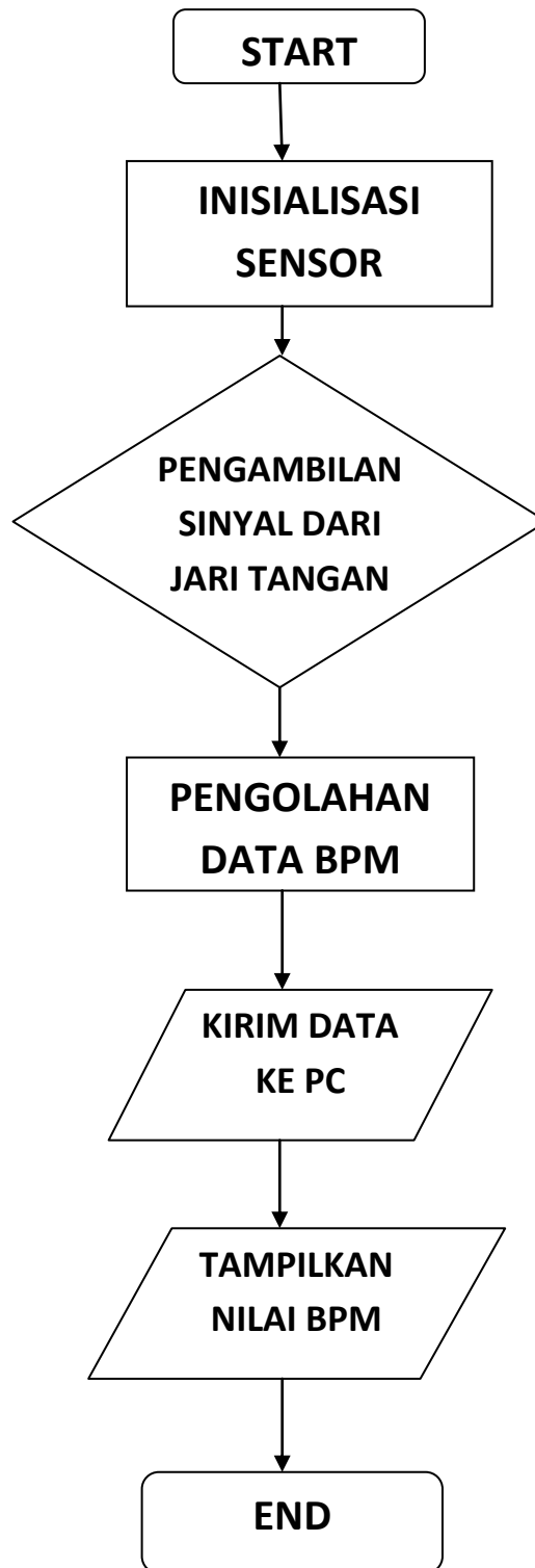
Gambar IV.5 Alur Kerja Sistem
