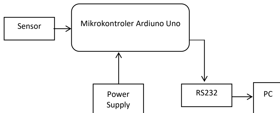
Gambar IV.2 Perancangan Perangkat Keras Secara Umum
