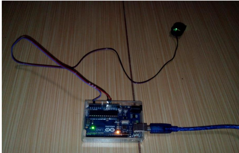
Gambar V.1 Rangkaian Sensor Pulsa dan Arduino Uno
