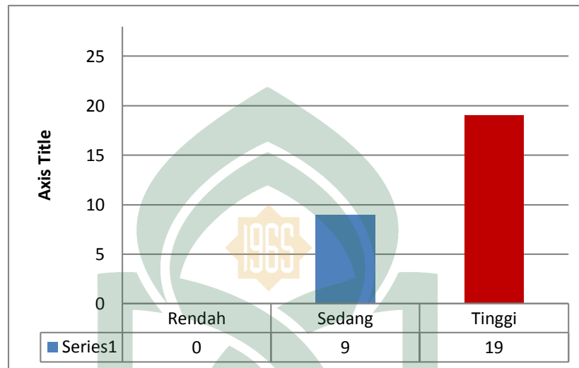
Gambar 4.1 : Histogram Kategori minat belajar sebelum diterapkan Metode Role Playing (Bermain Peran)
