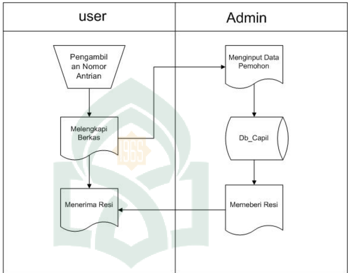
Gambar IV.2. Flowmap sistem yang diusulkan
