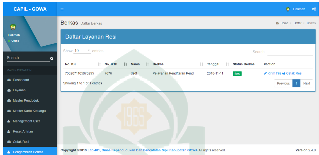
Gambar V.10 Daftar Berkas
