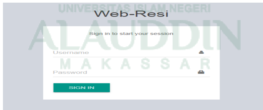
Gambar V.1 Halaman Login
