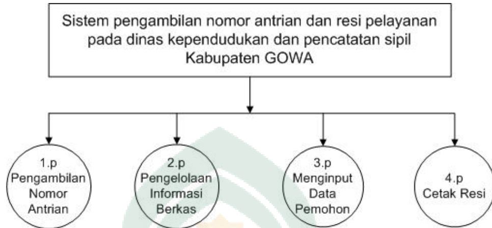
Gambar IV.4. Diagram Berjenjang
