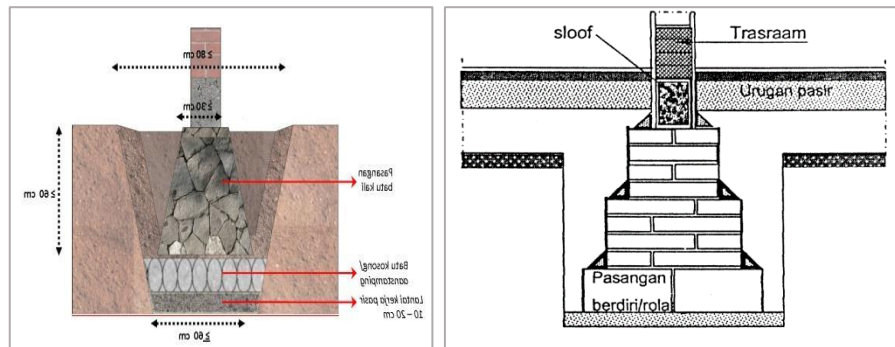
Gambar III.46. Pondasi Batu Kali dan Pondasi Batu Bata Sumber: Portal Unand, 2019
