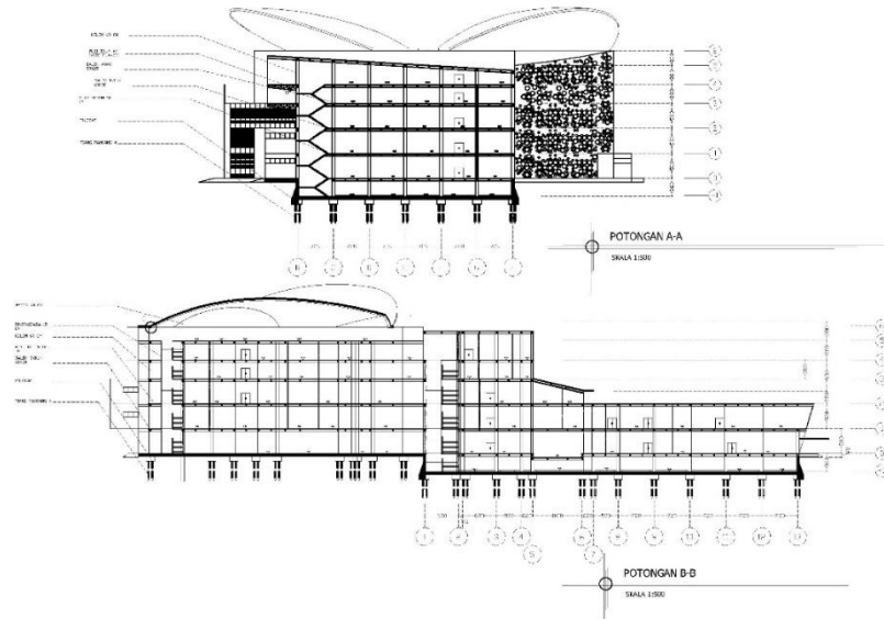
Gambar VI.8. Struktur Bangunan Sumber: Olah Desain, 2019
