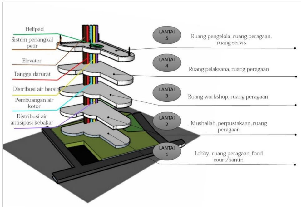
Gambar IV.10. Sistem Bentuk dan Pendukung Kelengkapan Bangunan Alternatif 2 Sumber: Olah Desain, 2019
