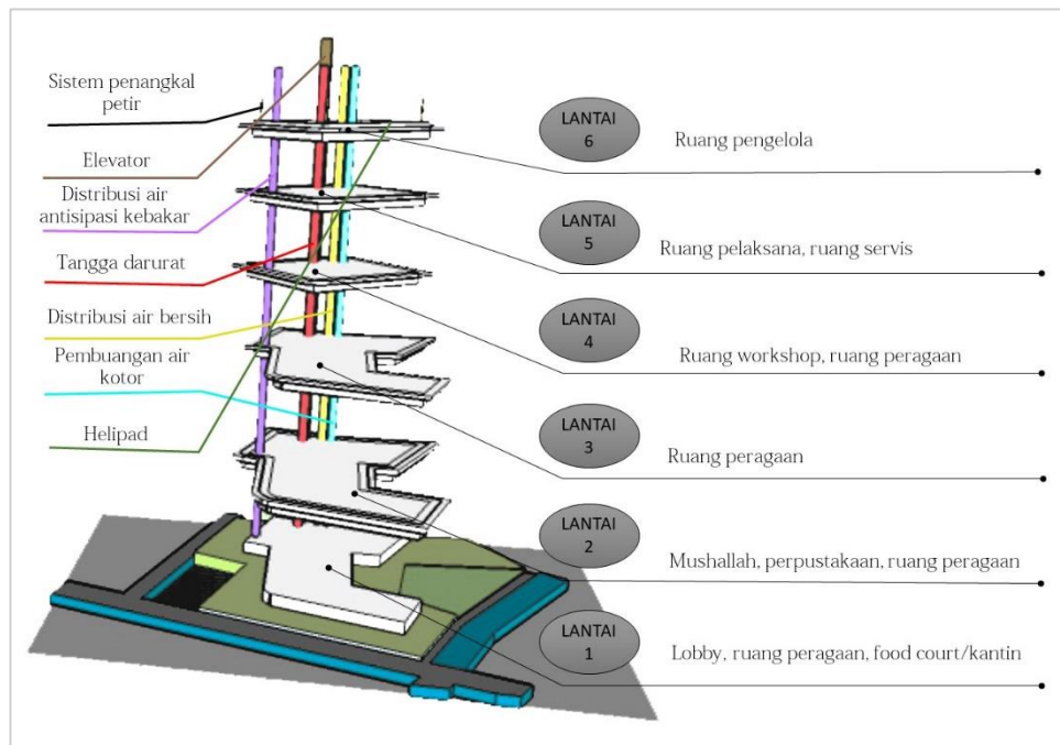
Gambar IV.8. Sistem Bentuk dan Pendukung Kelengkapan Bangunan 1 Sumber: Olah Desain, 2019
