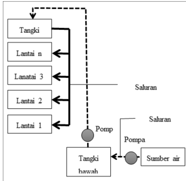
Gambar III.49. Bagan Sistem Distribusi Air Bersih Sumber: Sofyan dan Morimura, 1980
