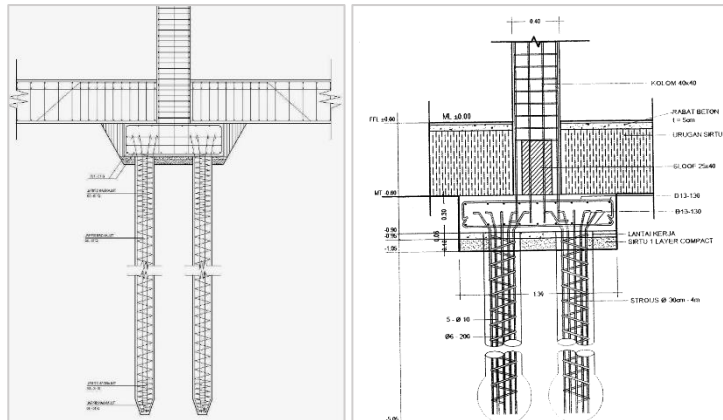
Gambar III.44. fondasi Tiang Pancang Sumber: Wordpress, 2019
