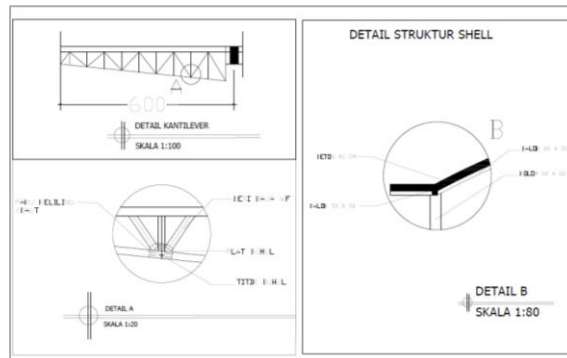
Gambar VI.9. Detail Struktur Bangunan Sumber: Olah Desain, 2019
