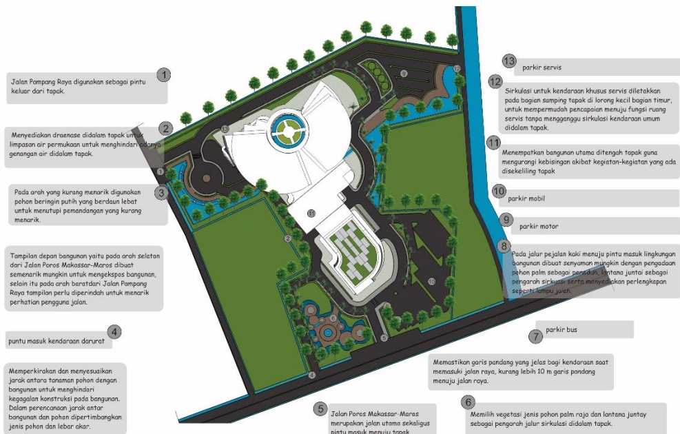
Gambar V.2. Desain Perencanaan Tapak Akhir Sumber: Olah Desain, 2019
