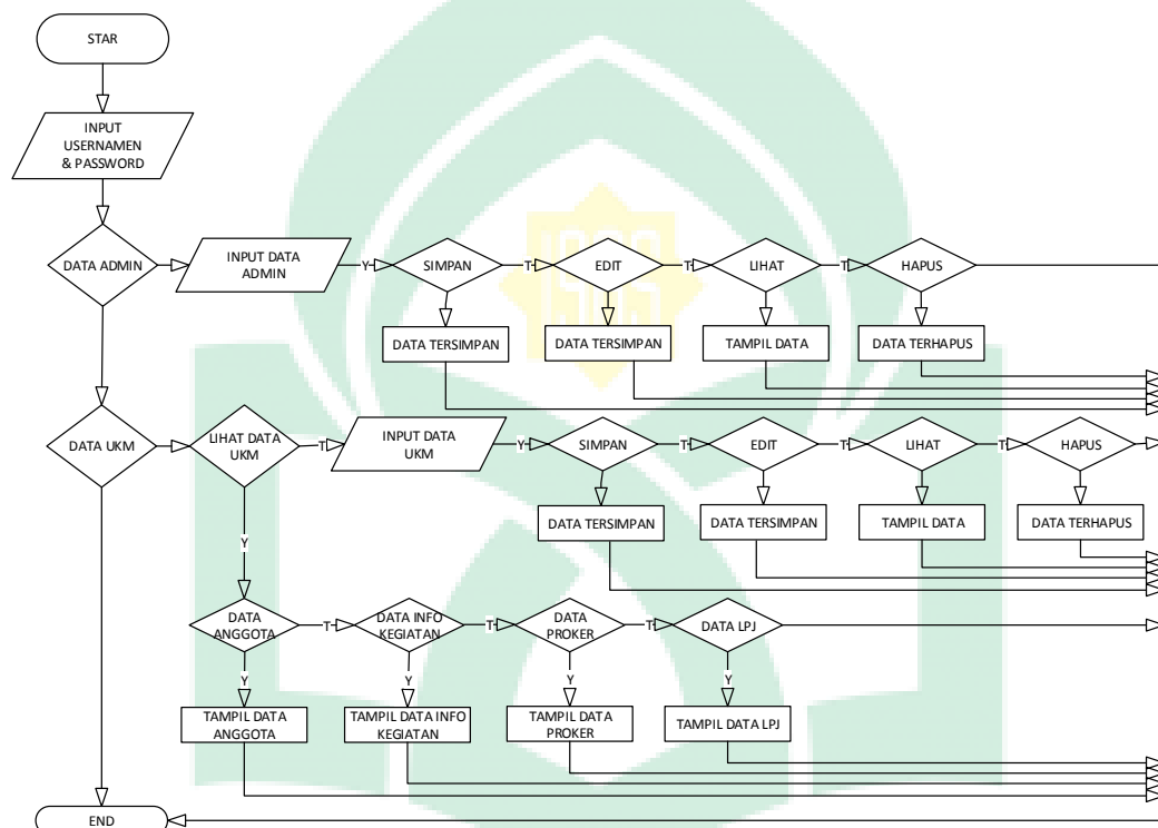
Gambar IV.18. Flowchart Admin Utama
