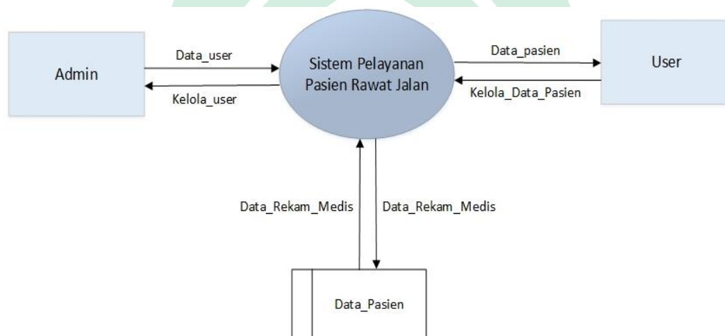
Gambar IV.8 Diagram Konteks
