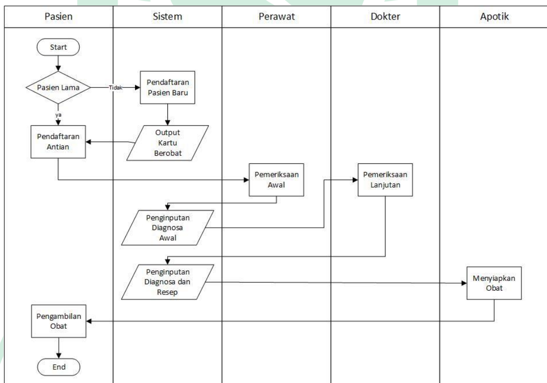
Gambar IV.2 Flowmap Sistem yang diusulkan.
