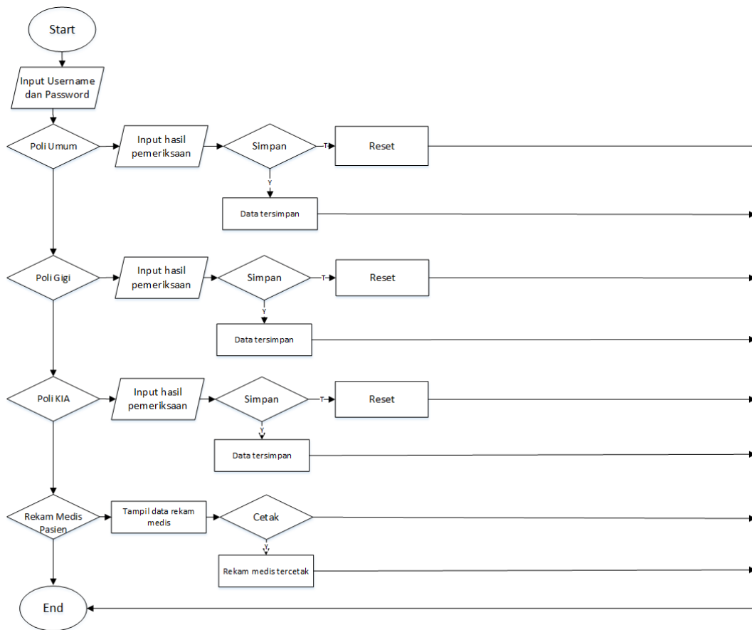
Gambar IV.6 Flowchart Dokter
