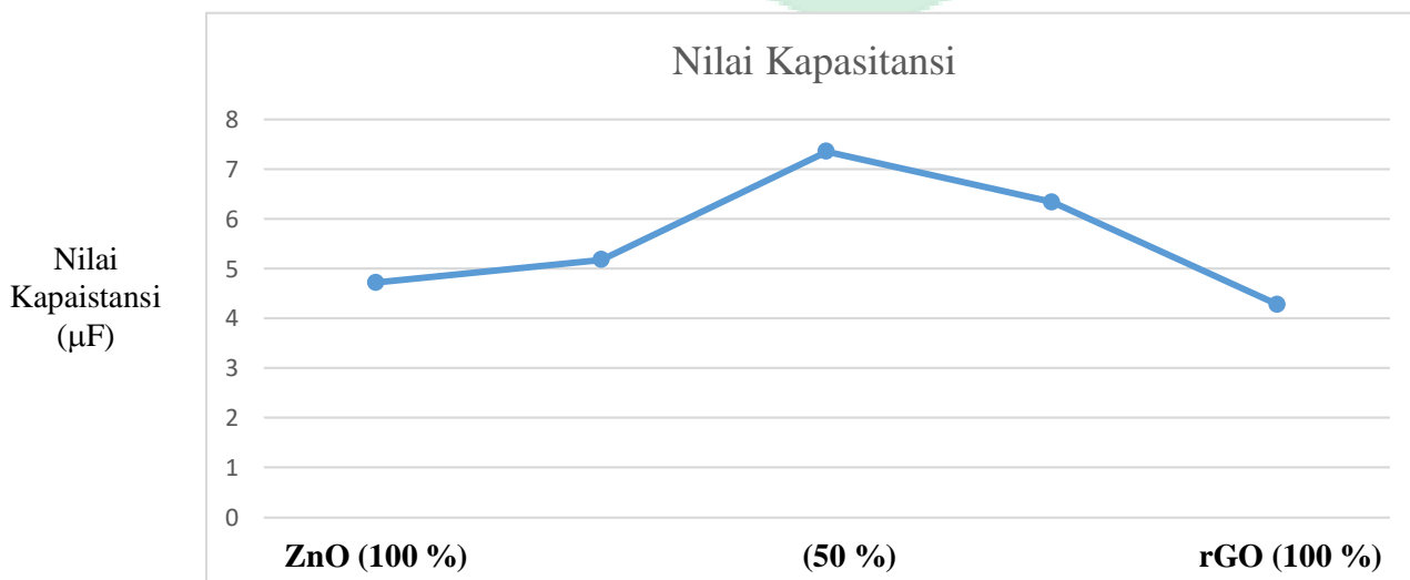
Gambar 4.9 Grafik uji kapasitansi rGO-ZnO
