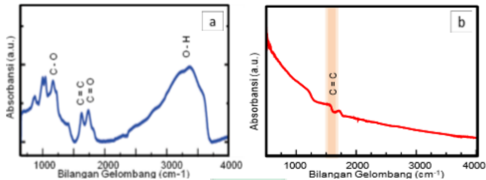
Gambar 2.7 Hasil karakterisasi Grafena menggunakan FTIR
