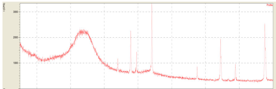
Gambar 4.8 Pola difraksi komposit rGO-ZnO
