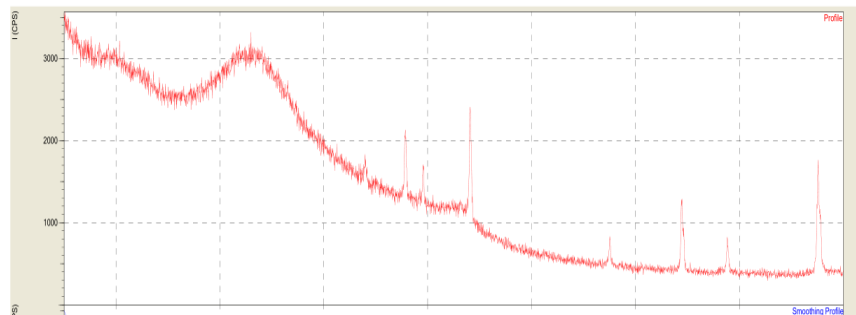
Gambar 4.7 Pola difraksi rGO
