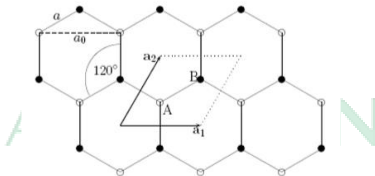
Gambar.2.2 Struktur Kisi Grafena
