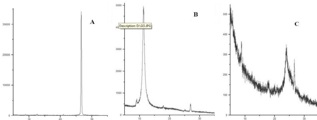
Gambar.2.5 Hasil XRD (A) grafit, (B) grafit oksida, dan (C) grafena (Taufantri, dkk., 2016)
