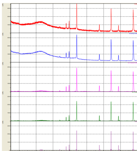
Gambar 4.1 Grafik XRD rGO
