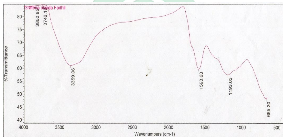
Gambar 4.5 Grafik FTIR rGO
