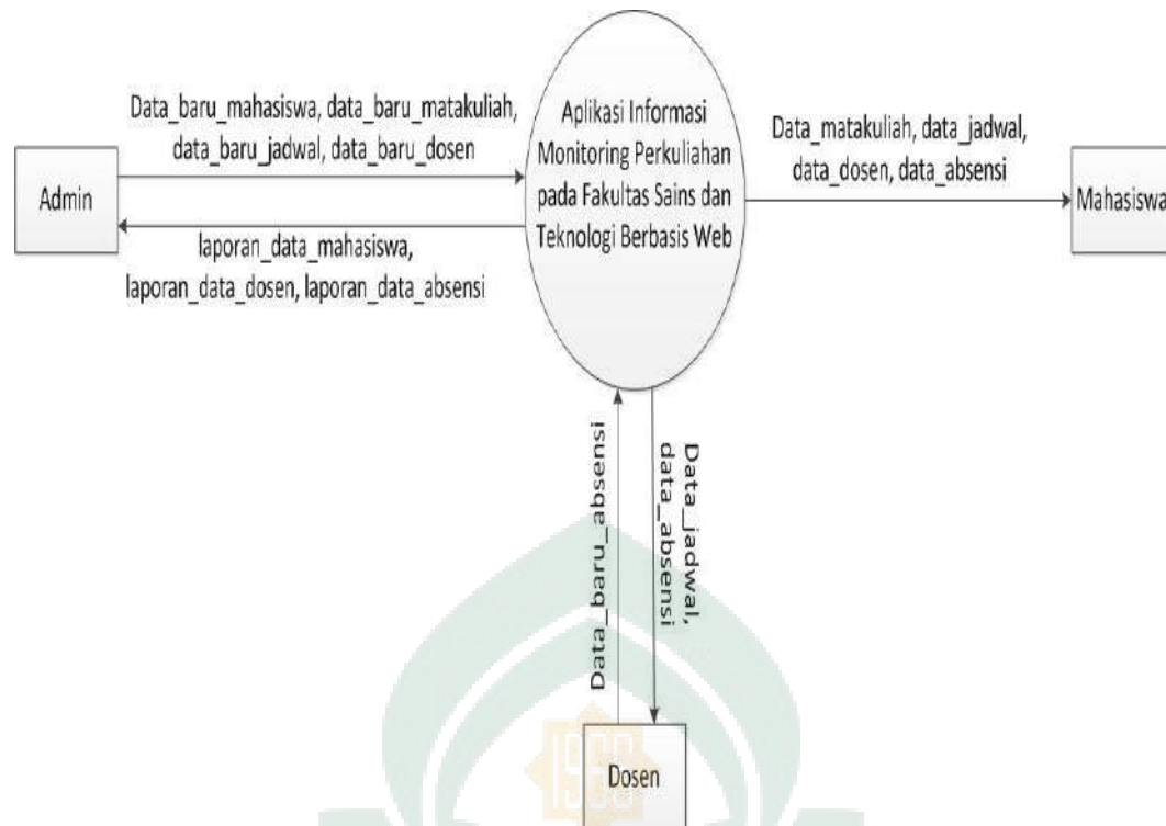
Gambar IV. 3. Diagram Konteks ( DFD Level 0)
