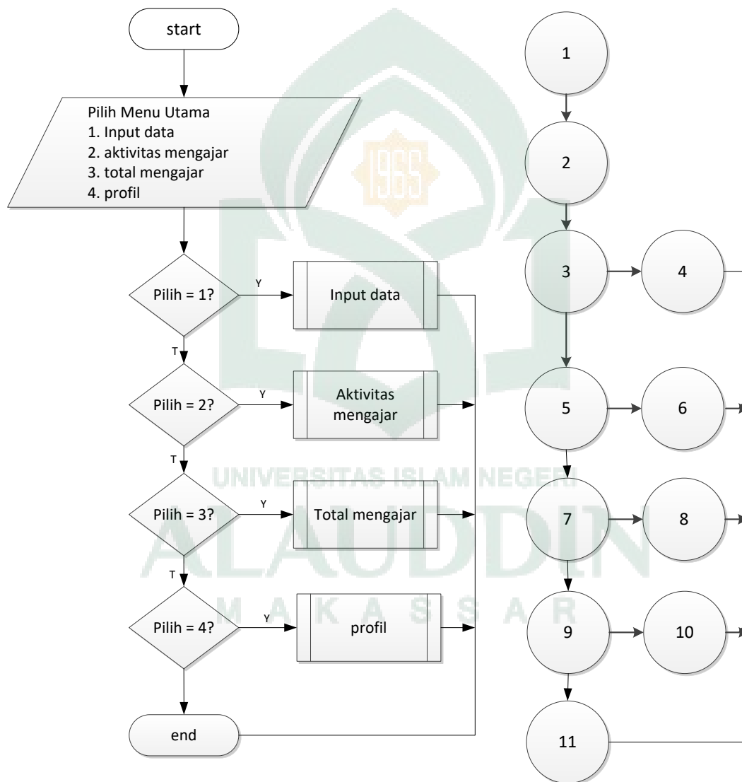
Gambar V. 9. Flowchart dan Flowgraph Menu Utama Dosen
