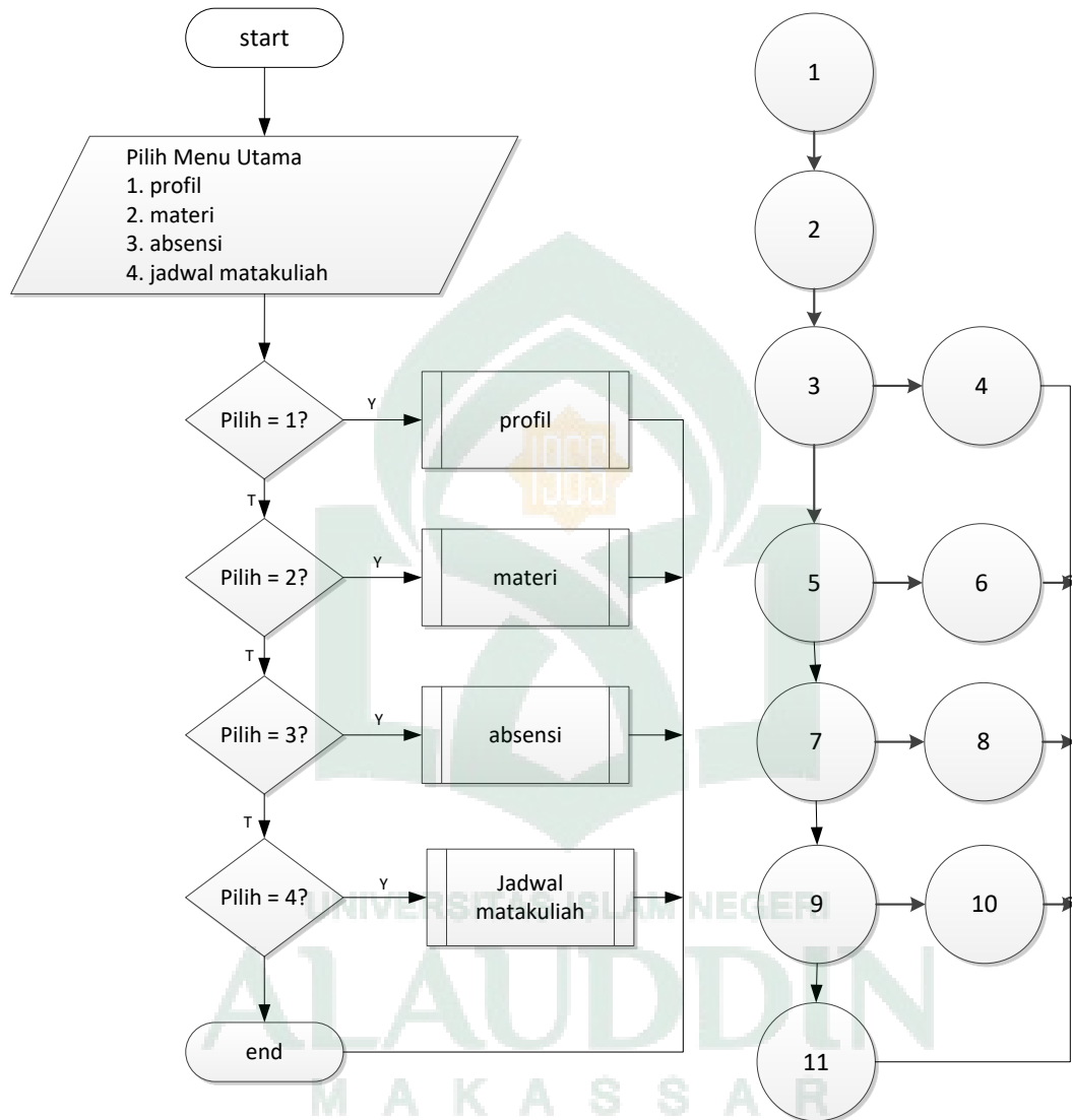
Gambar V. 11. Flowchart dan Flowgraph Halaman Utama Mahasiswa
