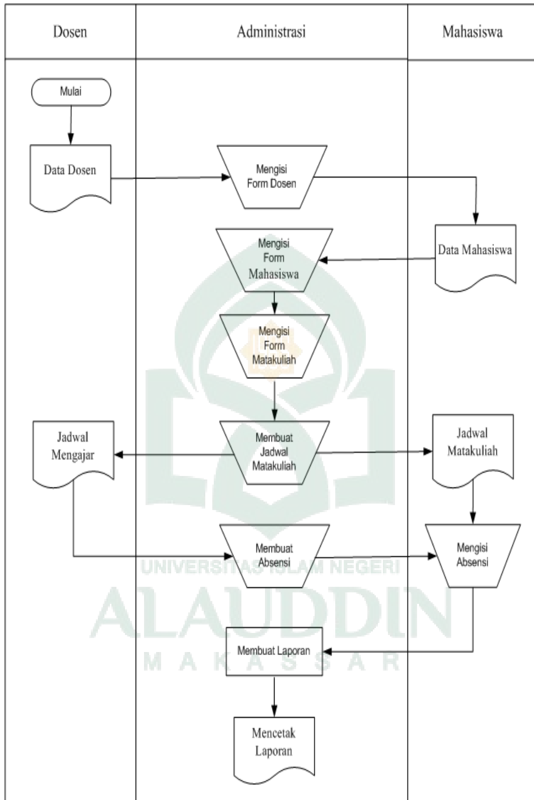
Gambar IV. 1. Proses Sistem yang Berjalan
