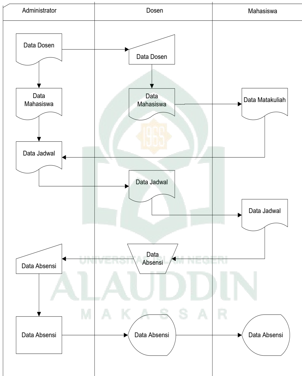
Gambar IV. 2. Proses Sistem yang Diusulkan
