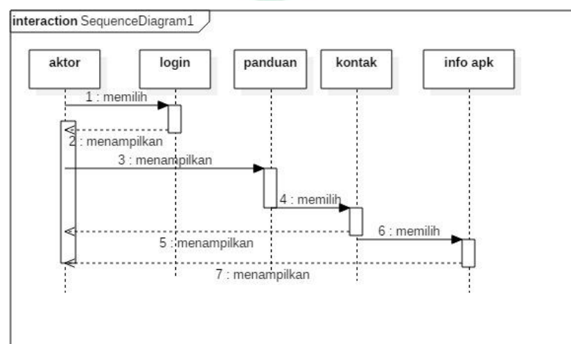
Gambar IV.6 Sequence Diagram pada login
