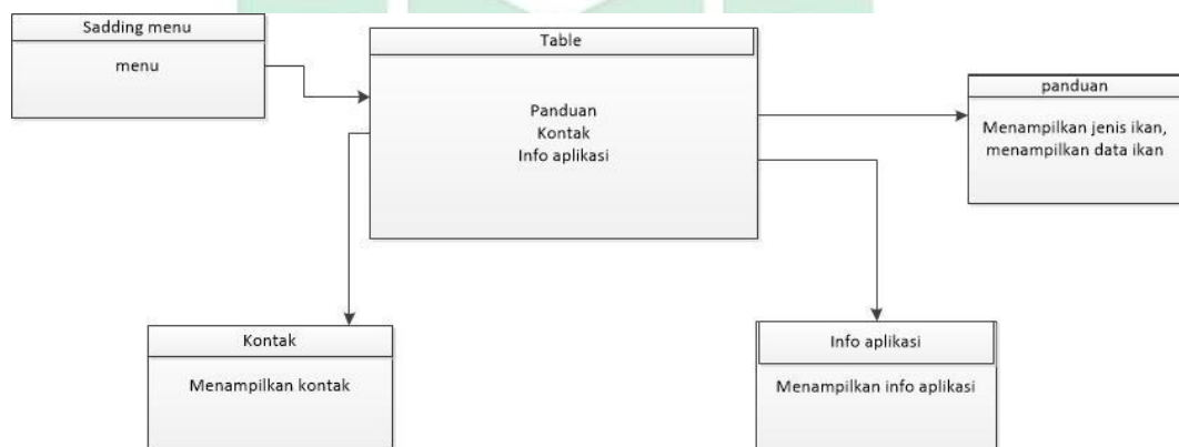
Gambar IV.4 Class Diagram Pengguna
