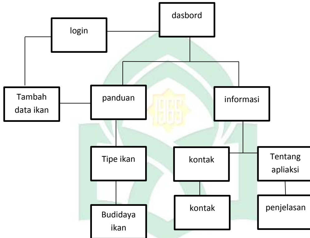
Gambar IV.14 Struktur Navigasi
