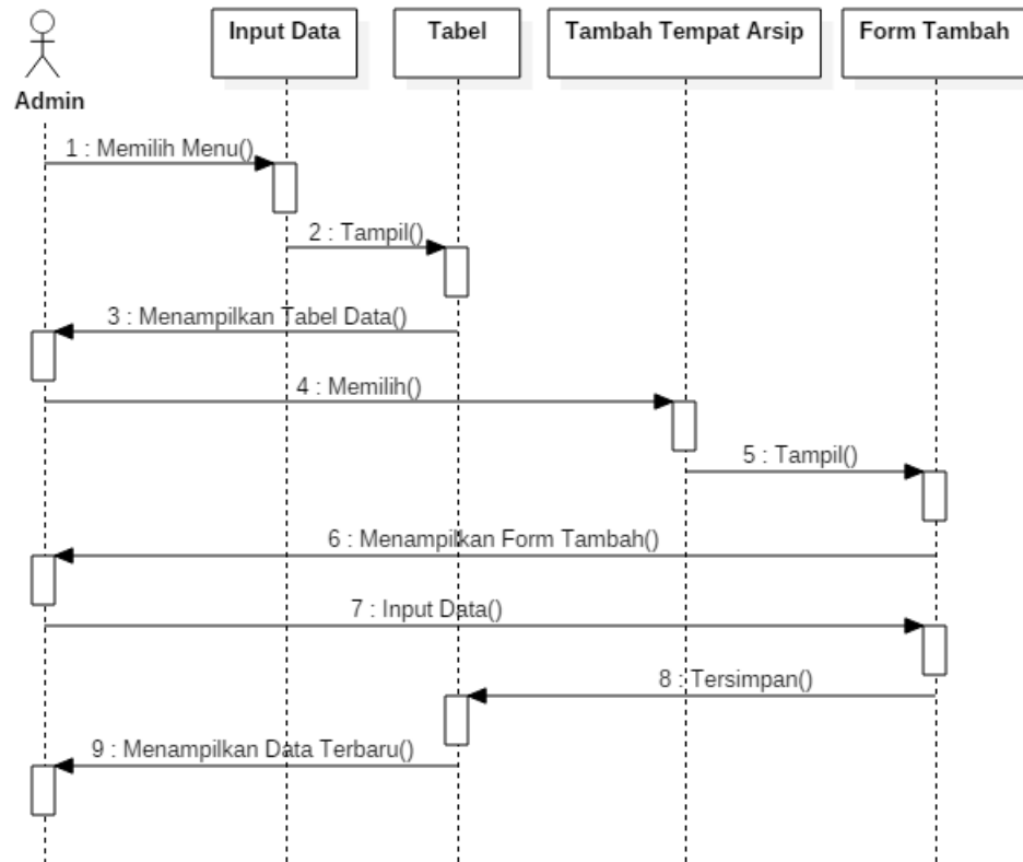
Gambar IV.8 Sequence diagram input data tempat arsip
