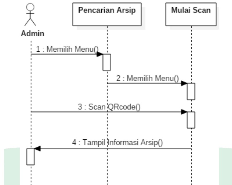
Gambar IV.5 Sequence Diagram pencarian untuk admin
