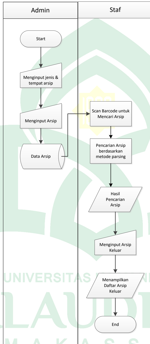
Gambar IV.2 Flowmap Diagram sistem yang diusulkan
