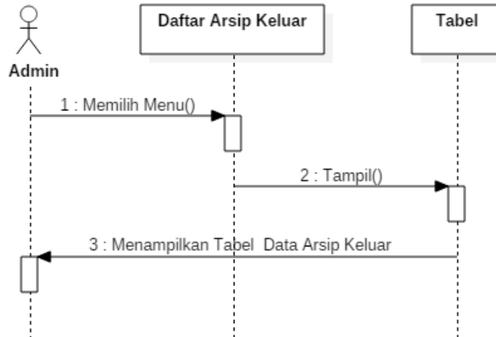
Gambar IV.12 Sequence diagram daftar arsip keluar untuk admin
