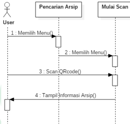
Gambar IV.6 Sequence Diagram pencarian arsip untuk user
