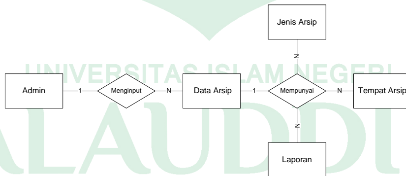
Gambar IV.13 ERD
