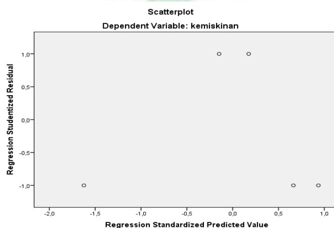
Gambar 1.3 : Uji Heteroskedastisitas
