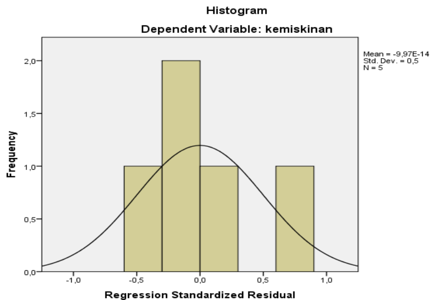
Gambar 1.1 : Grafik Histogram
