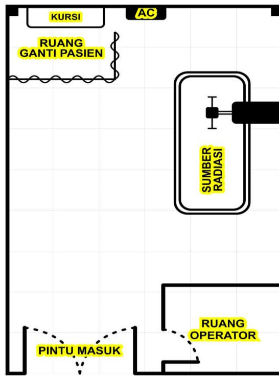
Gambar 2.8. Denah ruangan Pesawat sinar-X di RSUD Kota Makassar
