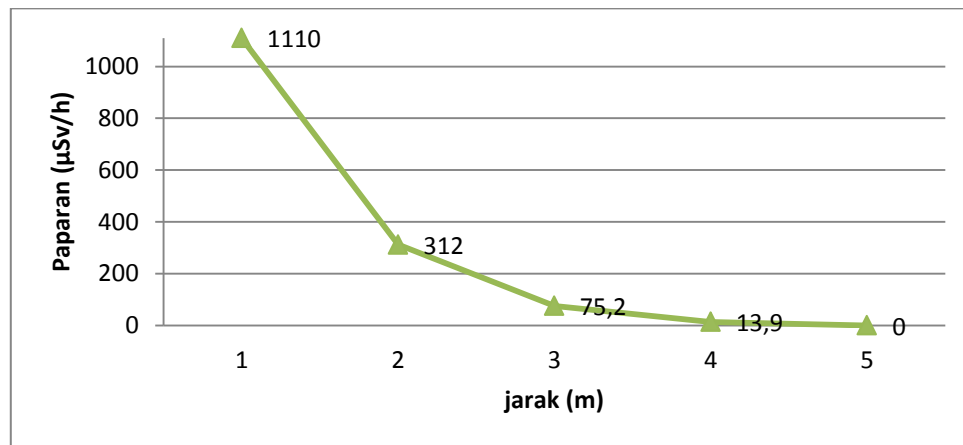
Gambar 4.3 : Grafik hasil pengukuran paparan radiasi sinar-X waktu 0,16 detik
