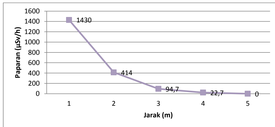
Gambar 4.4 : Grafik hasil pengukuran paparan radiasi sinar-X waktu 0,2 detik
