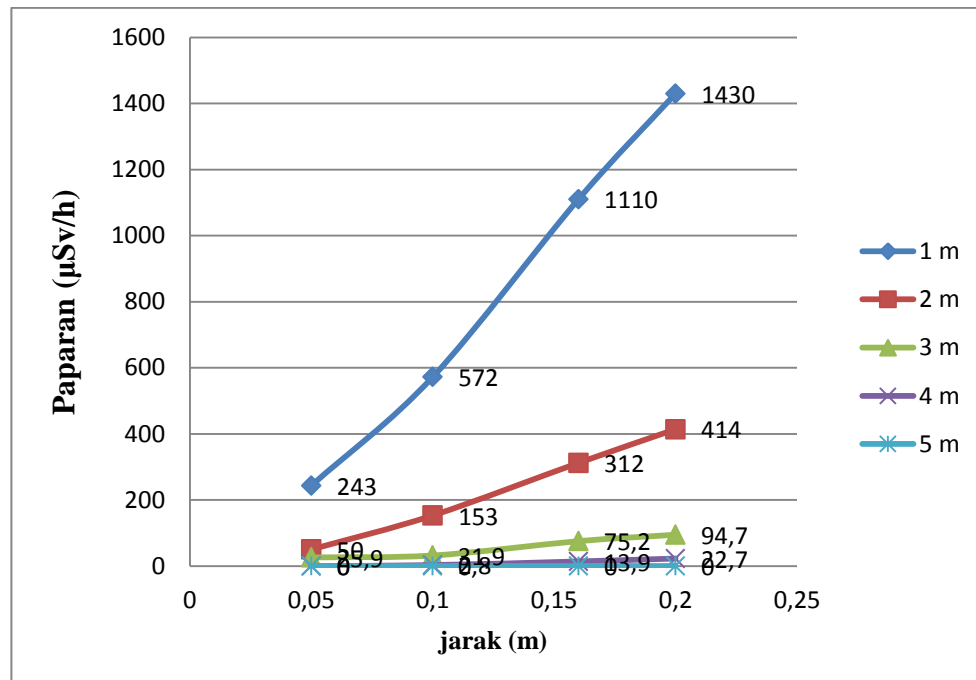
Gambar 4.5 Grafik pengaruh waktu paparan terhadap nilai dosis paparan radiasi
