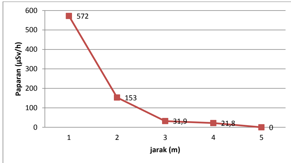
Gambar 4.2 : Grafik hasil pengukuran paparan radiasi sinar-X waktu 0,1 detik
