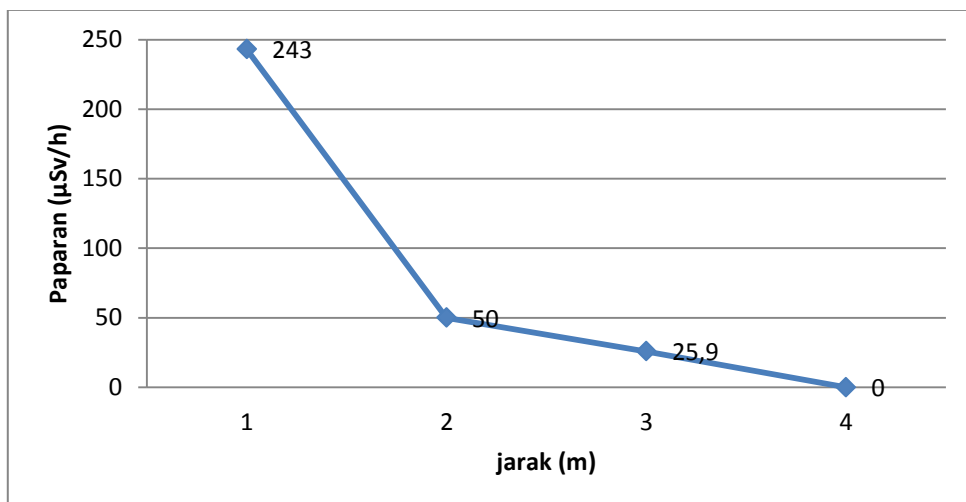
Gambar 4.1 : Grafik hasil pengukuran paparan radiasi sinar-X waktu 0,05 detik
