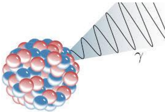
Gambar 2.3. Peluruhan sinar gamma sumber : Wikipedia.com 2019
