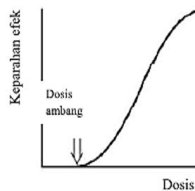
Gambar 2.6 Efek Deterministik Radiasi Sumber : Eri Hiswara 2015
