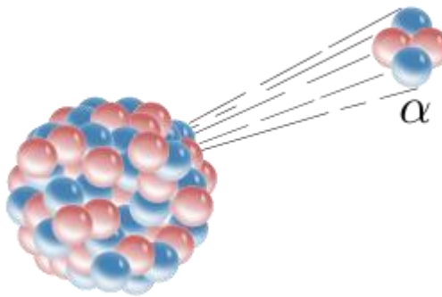
Gambar 2.1. Peluruhan sinar alfa sumber : Wikipedia.com 2019
