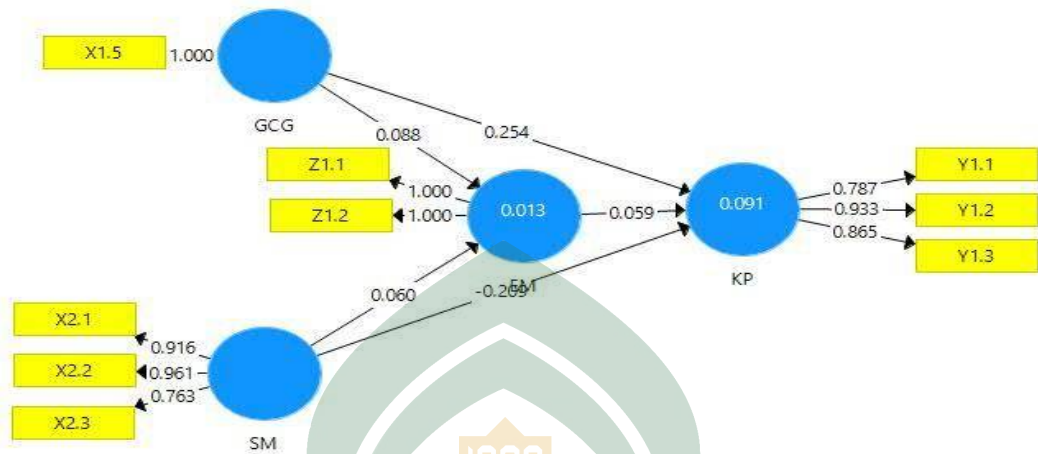
Gambar 4.2_ Outer Model Kedua
