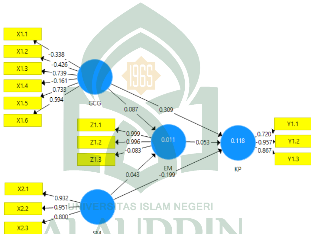
Gambar 4.1_Outer Model Pertama
