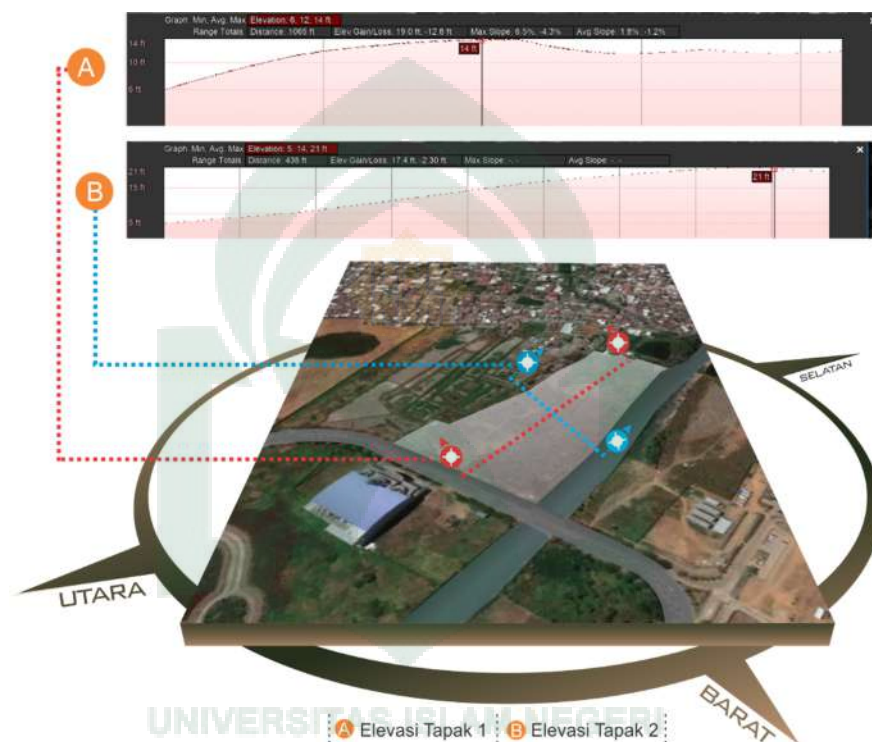
Gambar III.6. Analisis Topografi (Sumber: Olah Data, 20 Januari 2019)
