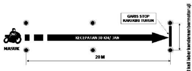
Gambar II.7. Uji Pengereman (Sumber: http://ditjenpp.kemenkumham.go.id/arsip/bn/2012/bn279-2012lamp.pdf , diakses pada tanggal 7 September 2018)
