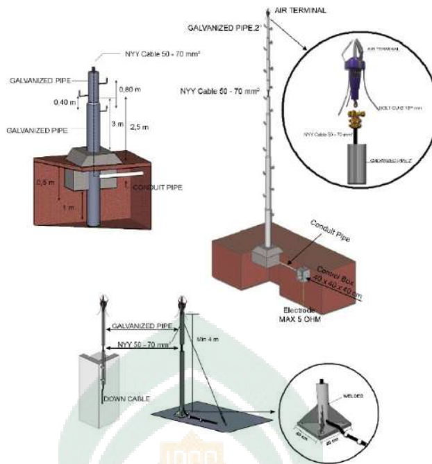
Gambar III.30. Sistem detail penangkal petir sistem thomas (Sumber: http://semarangpenangkalpetir.blogspot.com/ , diakses pada tanggal 30 Januari 2019)
