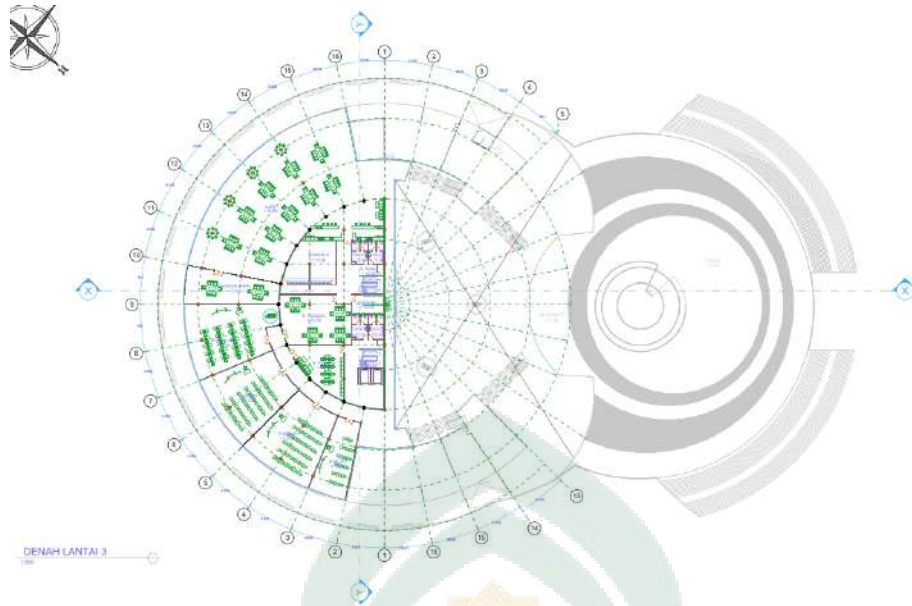
Gambar VI.5. Denah Lantai 3 Pusat Komunitas Motor Makassar (Sumber: Olah Desain, 2020)
