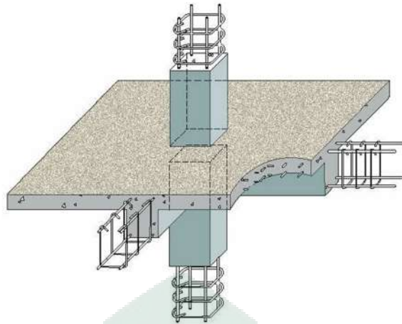
Gambar III.23. Struktur Tengah (Sumber: http://blog-oong.blogspot.com/2013/07/ , diakses pada tanggal 24 Januari 2019)
