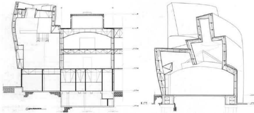
Gambar II.27. Potongan Museum Guggenheim Bilbao (Sumber: https://www.archdaily.com/422470/ad-classics-the-guggenheim-museum-bilbao-frank-gehry , diakses pada tanggal 11 oktober 2018)
