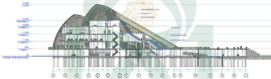
Gambar VI.11. Potongan X-X Pusat Komunitas Motor Makassar (Sumber: Olah Desain, 2020)
