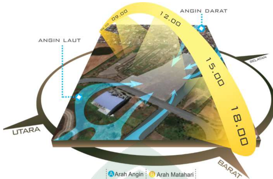
Gambar III.7. Analisis Iklim (Sumber: Olah Data, 20 Januari 2019)
