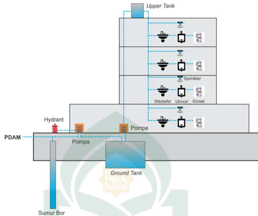
Gambar III.25. Analisis Sistem Jaringan Air Bersih (Sumber: Olah Data, 2019)
