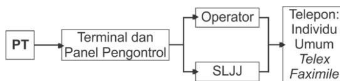
Gambar III.31. Jaringan Komunikasi Eksternal (Sumber: Olah Data, 2019)
