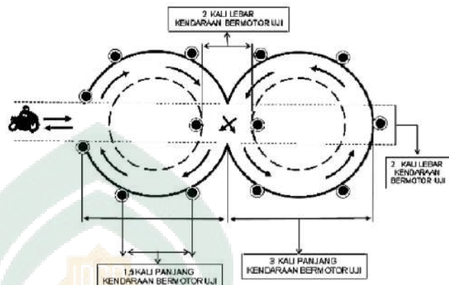
Gambar II.8. Uji Lintasan Angka Delapan (Sumber: http://ditjenpp.kemenkumham.go.id/arsip/bn/2012/bn279-2012lamp.pdf , diakses pada tanggal 7 September 2018)
