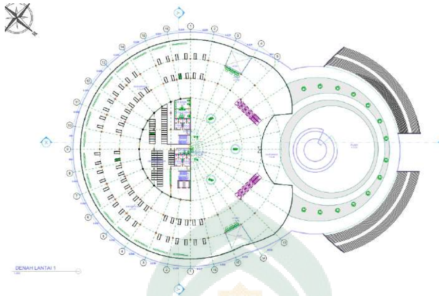
Gambar VI.3. Denah Lantai 1 Pusat Komunitas Motor Makassar (Sumber: Olah Desain, 2020)
