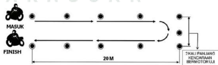
Gambar II.9. Uji Berbalik Arah (Sumber: http://ditjenpp.kemenkumham.go.id/arsip/bn/2012/bn279-2012lamp.pdf , diakses pada tanggal 7 September 2018)
