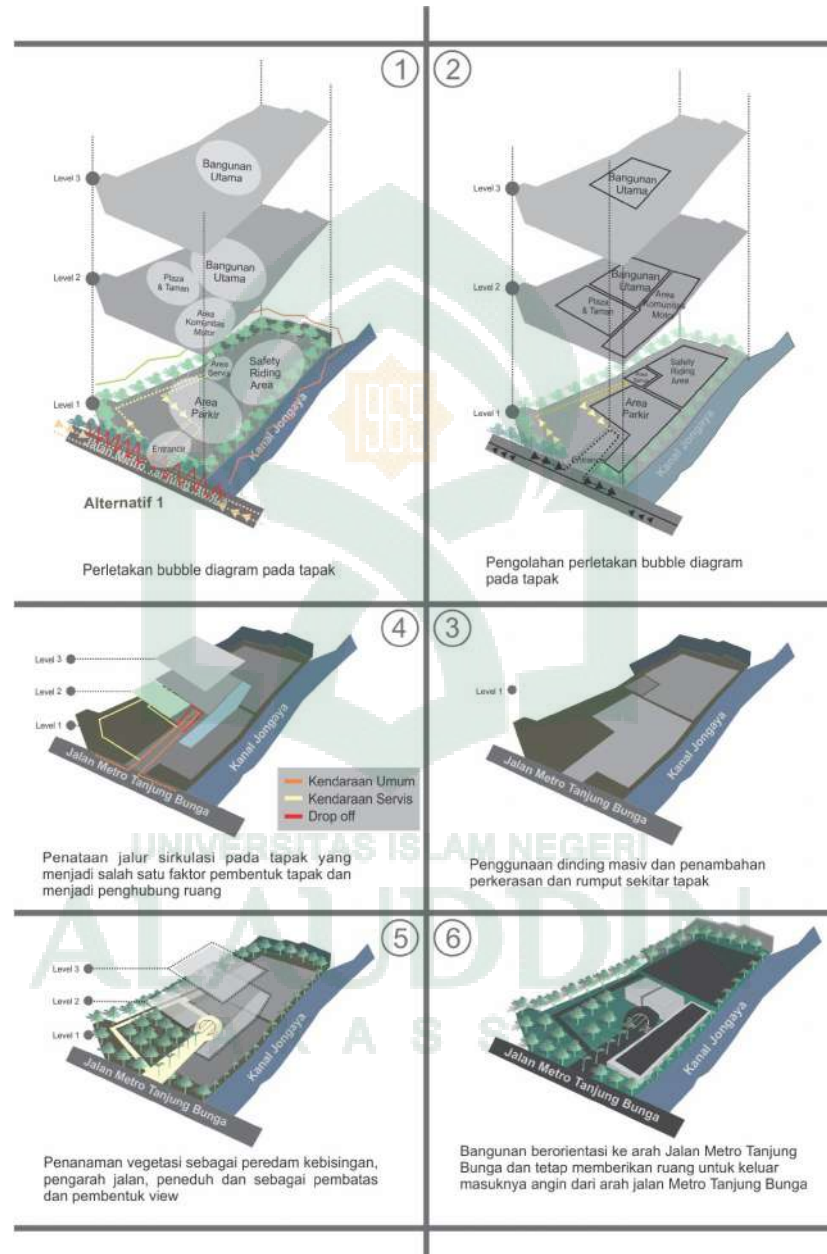
Gambar IV.4. Alternatif 1 Gagasan Pemrograman Ruang Hubungannya dengan Pengolahan Bentuk Tapak (Sumber: Olah Desain, 2019)
