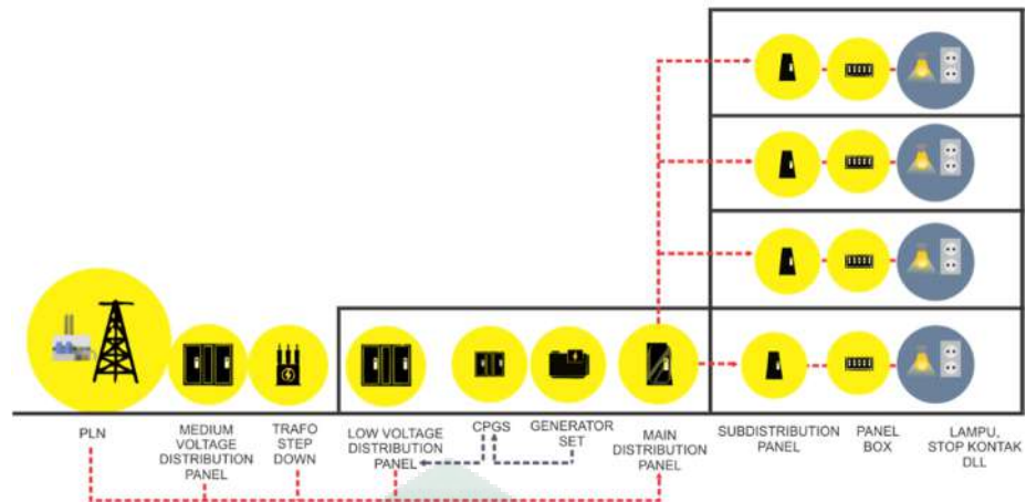
Gambar III.27. Analisis Sistem Jaringan Listrik (Sumber: Olah Data, 2019)
