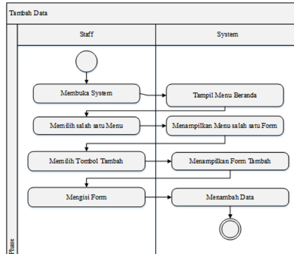
Gambar IV. 14 Aktiviti Diagram Tambah Data
