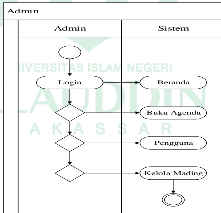
Gambar IV. 17 Aktivitas Diagram Menu Admin
