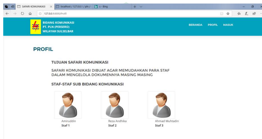
Gambar V.32 Halaman Profil
