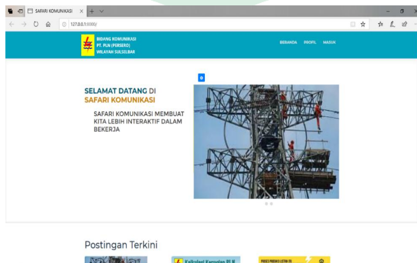
Gambar V. 31 Halaman Utama
