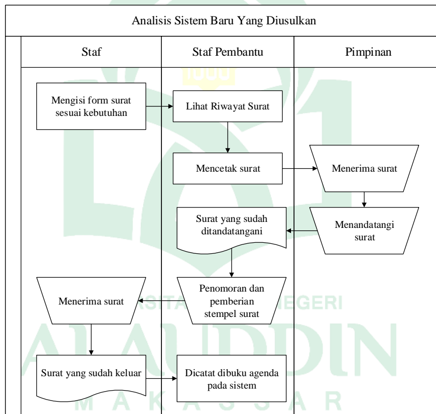
Gambar IV.3 Flowmap Diagram Yang Diusulkan
