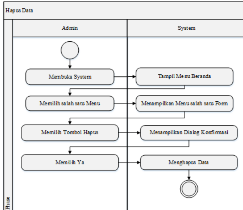
Gambar IV. 16 Aktivitas Diagram Hapus data
