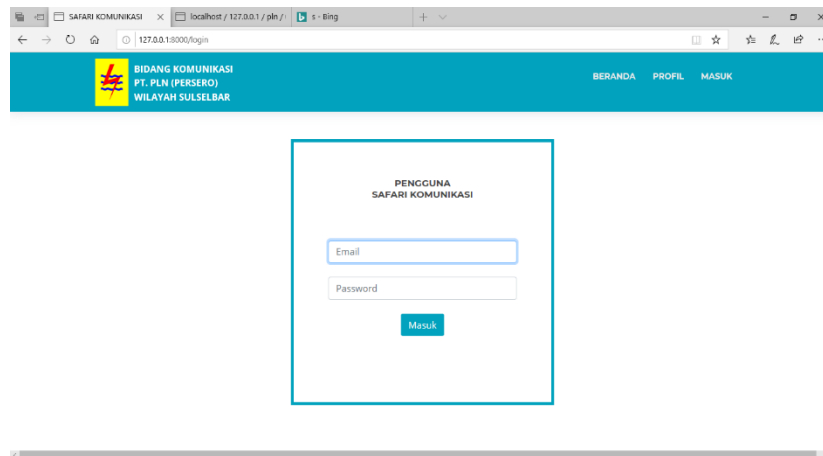
Gambar V.33 Halaman Login
