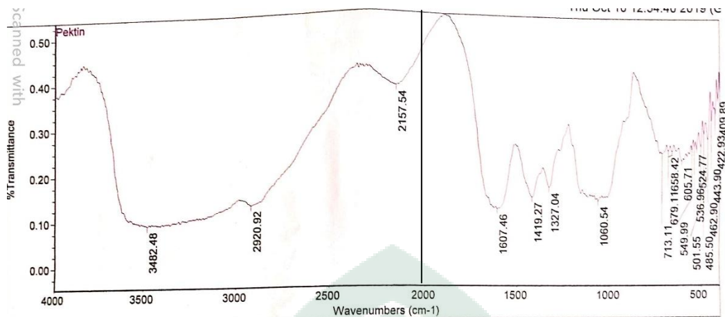
Gambar 4.1 Spektrum FTIR Pektin Kulit Pisang Ambon
