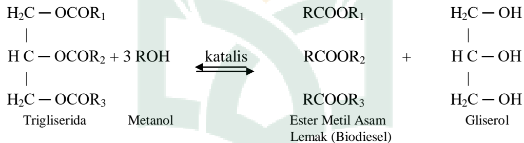
Gambar 2.3 Reaksi Pembentukan Gliserol
