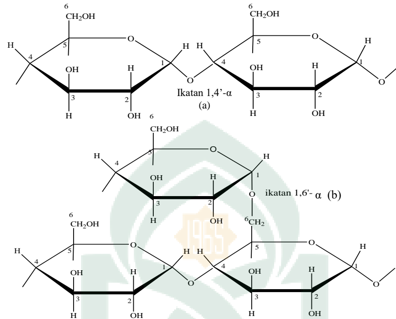
Gambar 2.5 Struktur Amilosa (a) dan Amilopektin (b)
