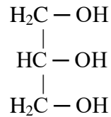
Gambar 2.4 Rumus Struktur Gliserol
