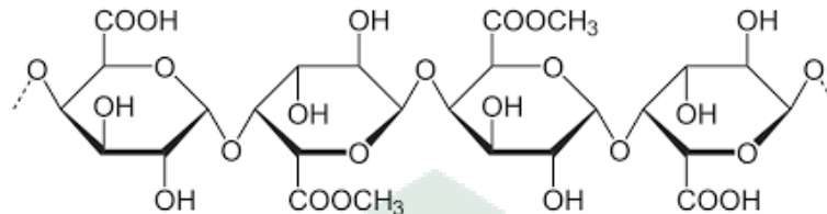
Gambar 2.2 Struktur Pektin
