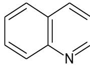
Gambar 2.5 Struktur Alkaloid
