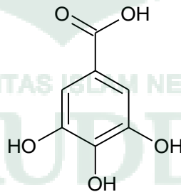
Gambar 2.6 Struktur Tanin
