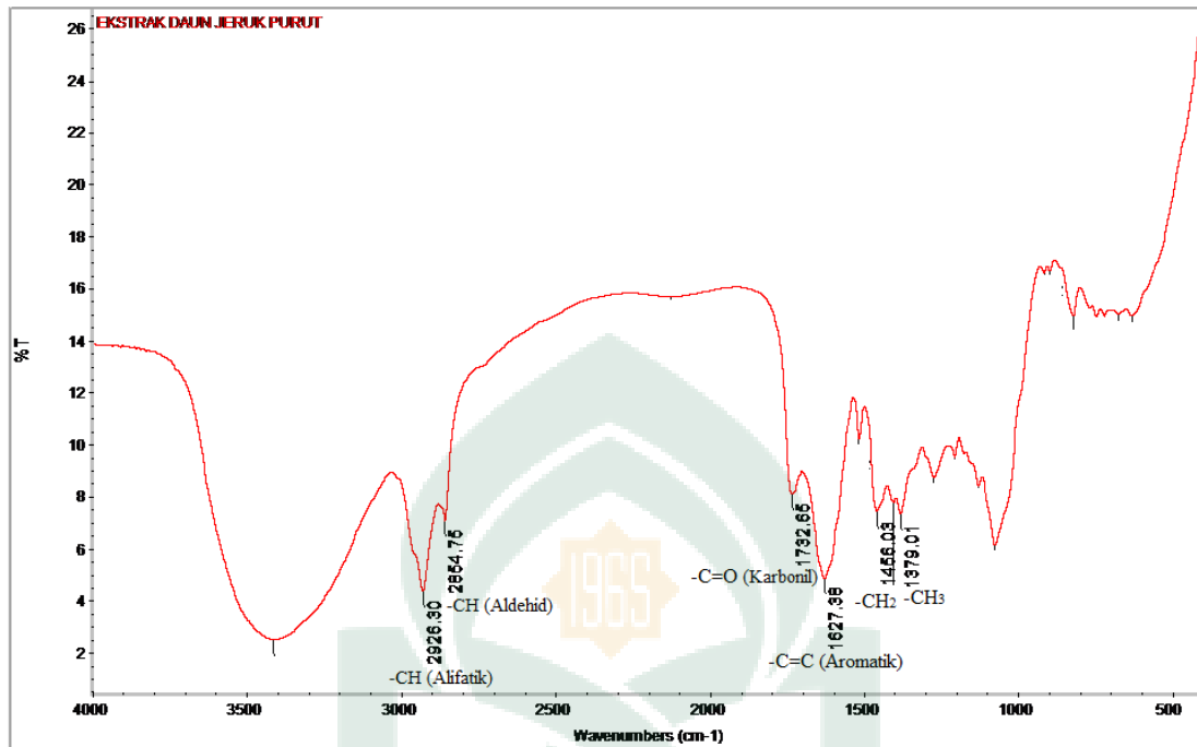
Gambar 4.1 Spektrum FTIR Ekstrak Daun Jeruk Purut ( Citrus hystrix DC)
