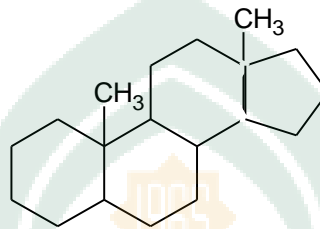
Gambar 2.7 Struktur Steroid
