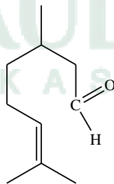
Gambar 2.3 Struktur Sitronellal
