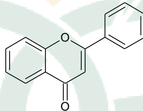
Gambar 2.4 Struktur Flavonoid
