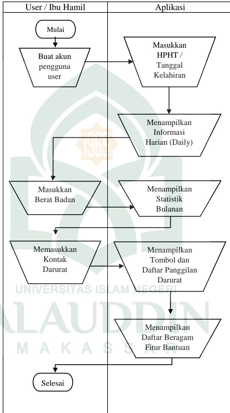
Gambar IV.2 Diagram Flowmap Sistem Yang Diusulkan
