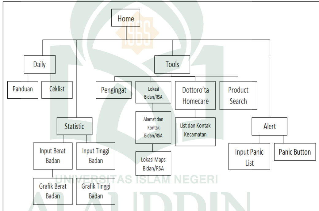
Gambar IV.15 Struktur Navigasi
