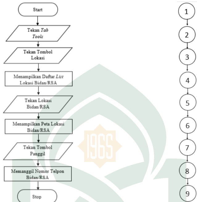
Gambar V.14 Flowchart dan Flowgraph Fitur Lokasi Bidan/RSA
