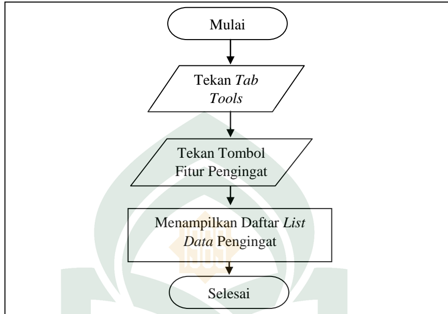
Gambar IV.11 Flowchart Fitur Pengingat
