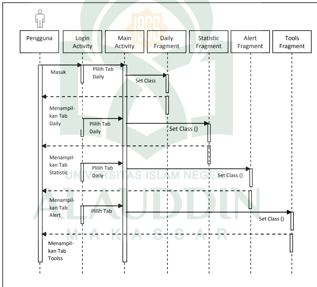
Gambar IV.5 Sequence Diagram Menu Aplikasi
