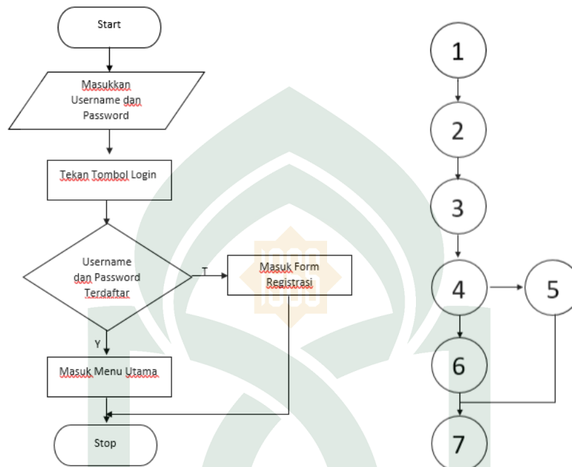
Gambar V.8 Flowchart dan Flowgraph Menu Login
