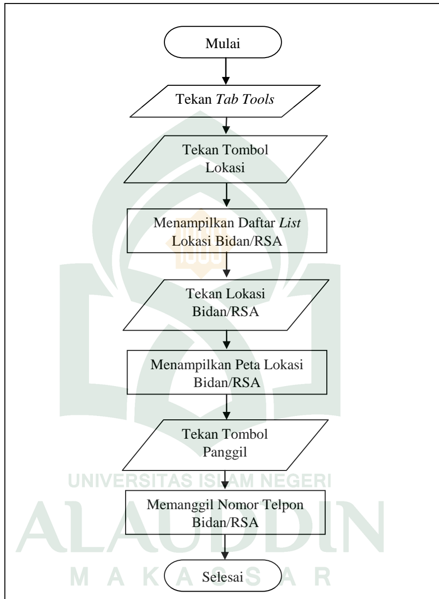
Gambar IV.13 Flowchart Fitur Lokasi Bidan/RSA
