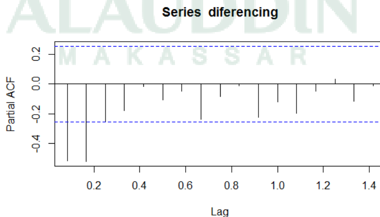
Gambar 4.6 Plot PACF Data Penggunaan Air
