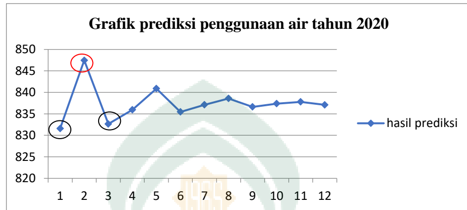
Gambar 4.7 Grafik hasil prediksi penggunaan air tahun 2020
