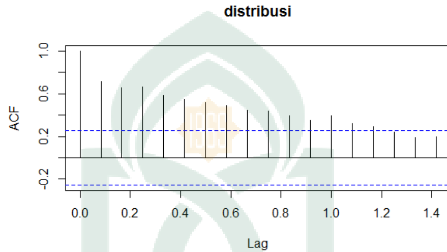
Gambar 4.2 Plot ACF Data Penggunaan Air
