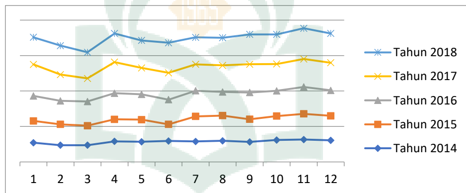
Gambar 4.1 Grafik Penggunaan Air di Kabupaten Gowa
