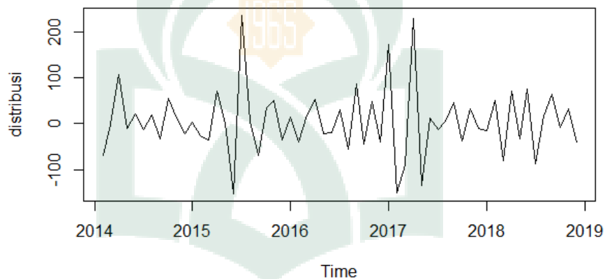
Gambar 4.4 Plot Data Penggunaan Air Setelah Differencing Non Musiman
