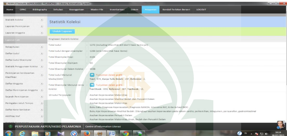
Gambar 12. Modul pelaporan
