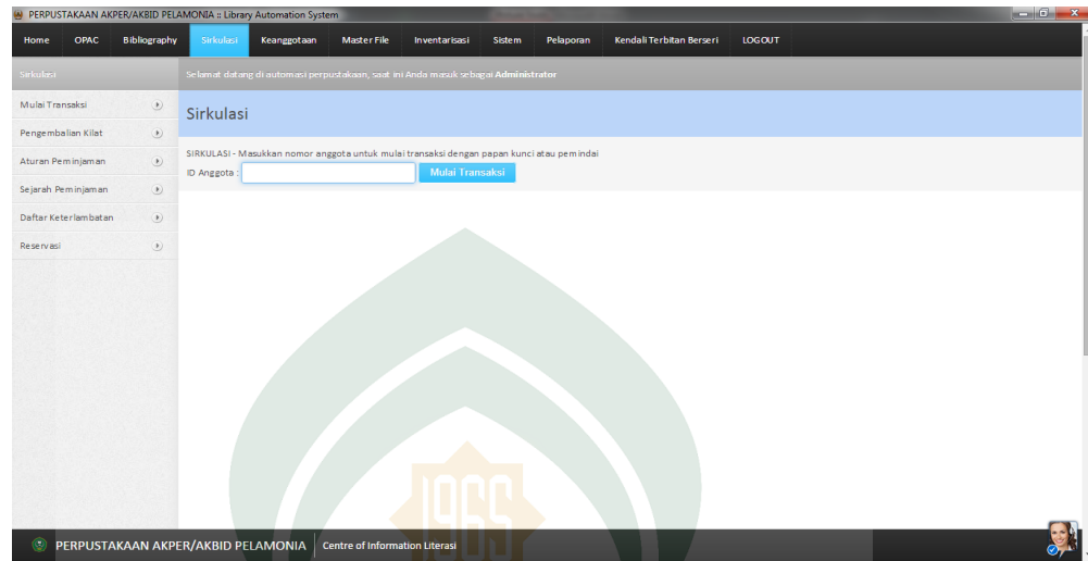
Gambar 6. Modul sirkulasi
