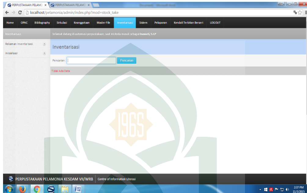
Gambar 11. Modul inventarisasi
