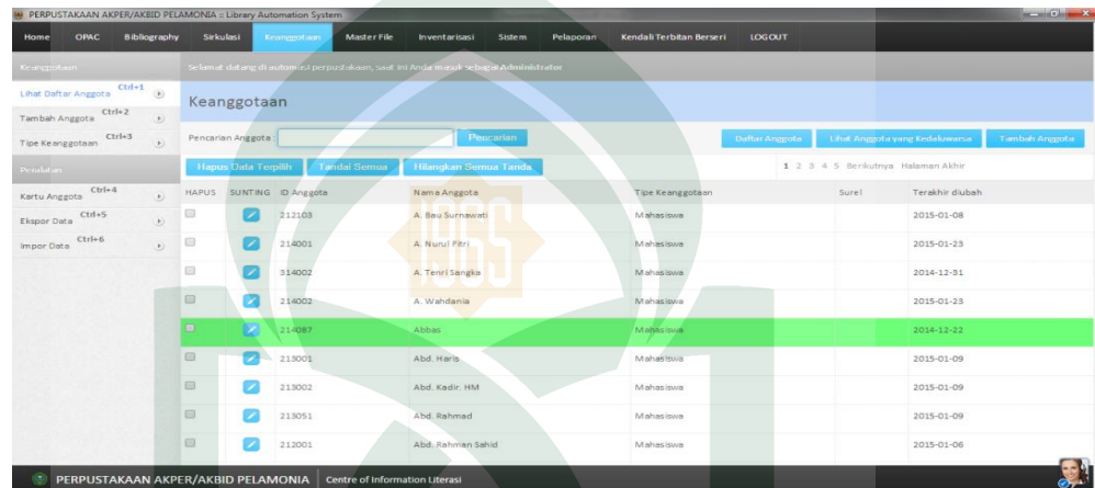
Gambar 8. Modul keanggotaan
