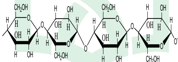
Gambar 2.2 Struktur Selulosa (Sumber: Baharuddin, dkk., 2016: 2)
