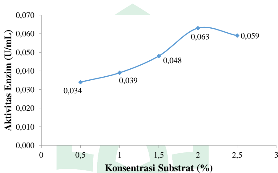
Gambar 4.4 Pengaruh Konsentrasi Substrat terhadap Aktivitas Enzim Selulase
