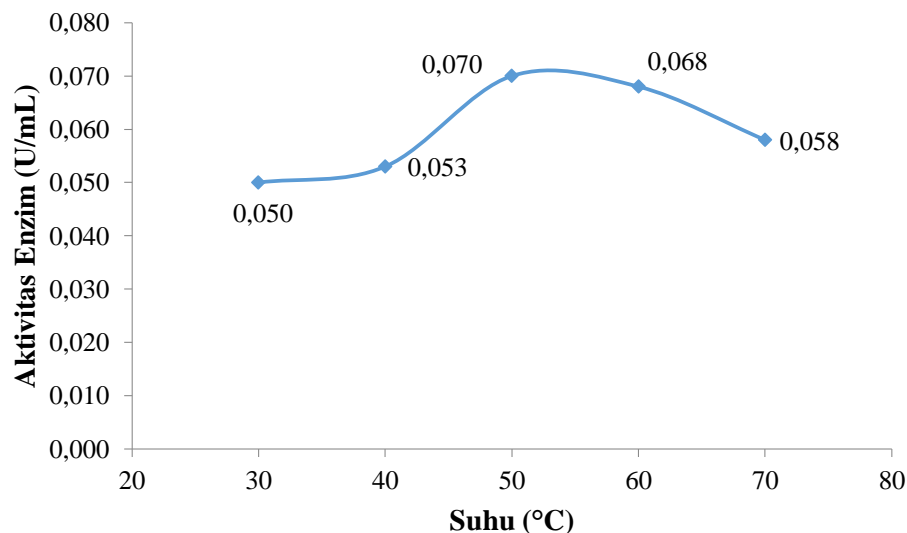
Gambar 4.2 Pengaruh Suhu Terhadap Aktivitas Enzim Selulase
