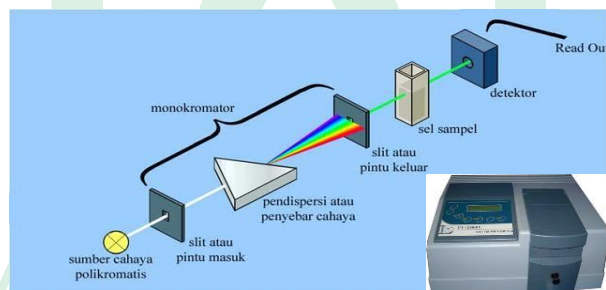
Gambar 2.4 Spektrofotometer UV-Vis (Sumber: Azizah, 2017: 18)
