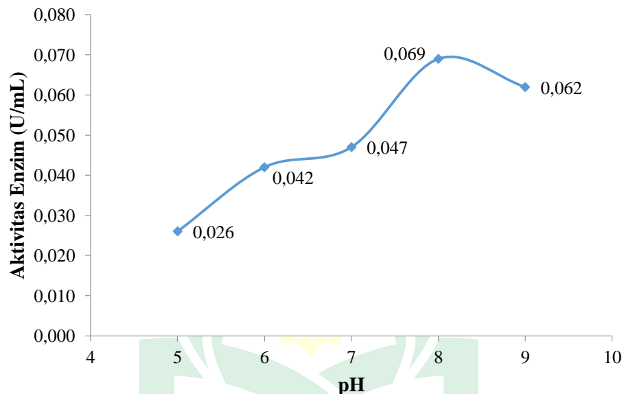
Gambar 4.3 Pengaruh pH terhadap Aktivitas Enzim Selulase
