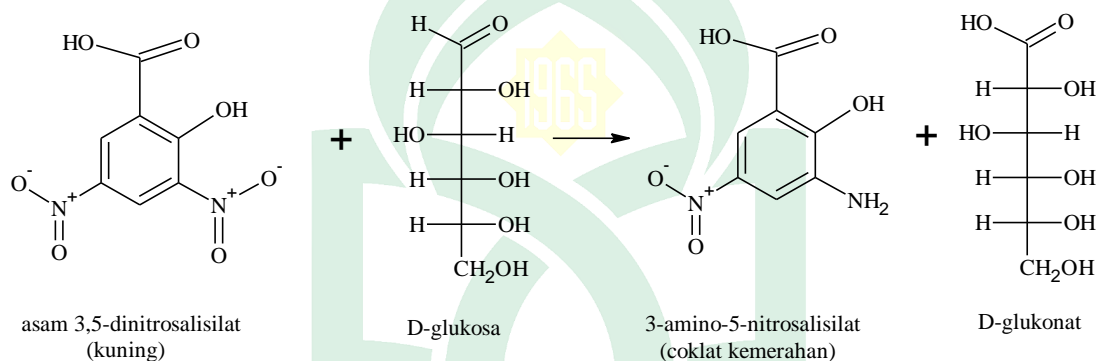
Gambar 4.1 Reaksi asam dinitrosalisilat (DNS) dengan glukosa
