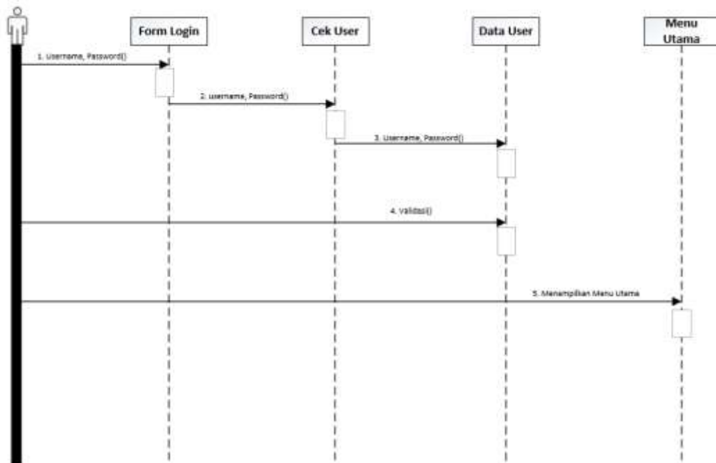
Gambar IV. 5 Sequence Diagram Untuk Login
