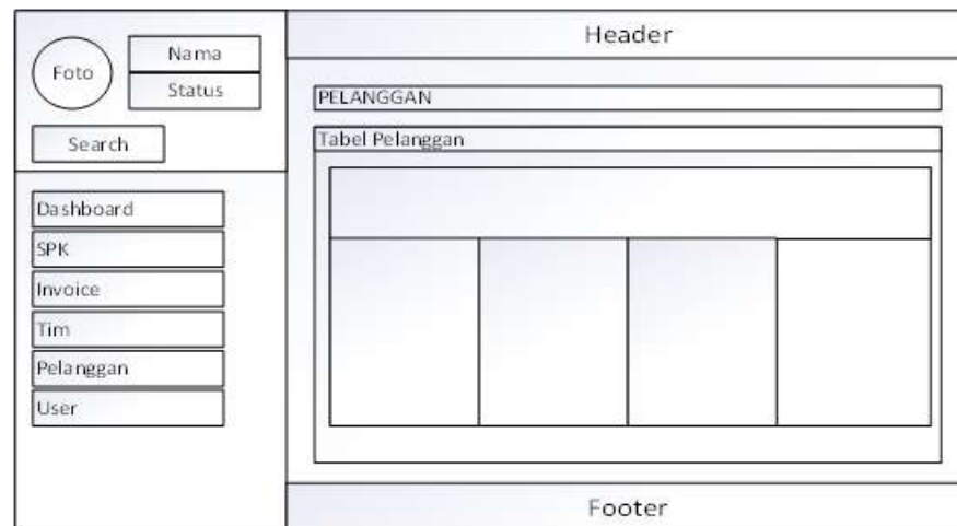
Gambar IV. 14 Antarmuka Pelanggan
