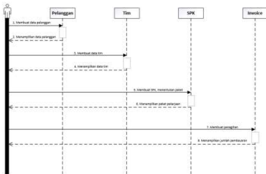
Gambar IV. 6 Sequence Diagram Membuat Data
