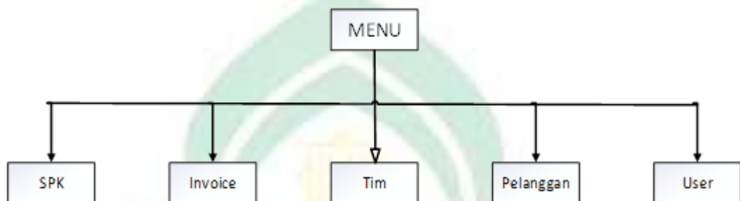
Gambar IV. 8 Struktur Navigasi
