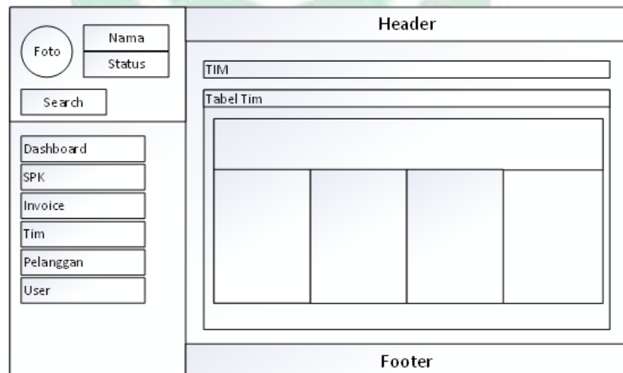
Gambar IV. 13 Antarmuka Tim
