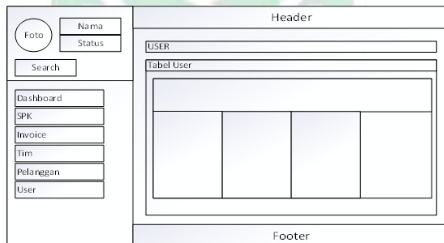
Gambar IV. 15 Antarmuka User
