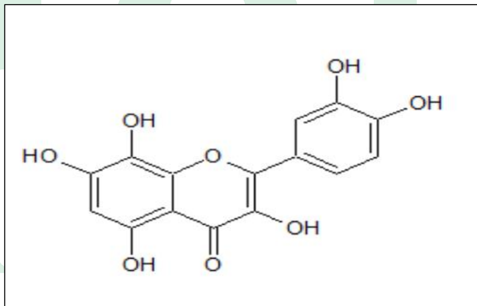
Gambar 2.3 Struktur Kuersetin
