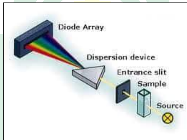
Gambar 2.5 Proses Penyerapan Sinar UV-Vis Oleh Larutan Sampel Dalam Kuvet
