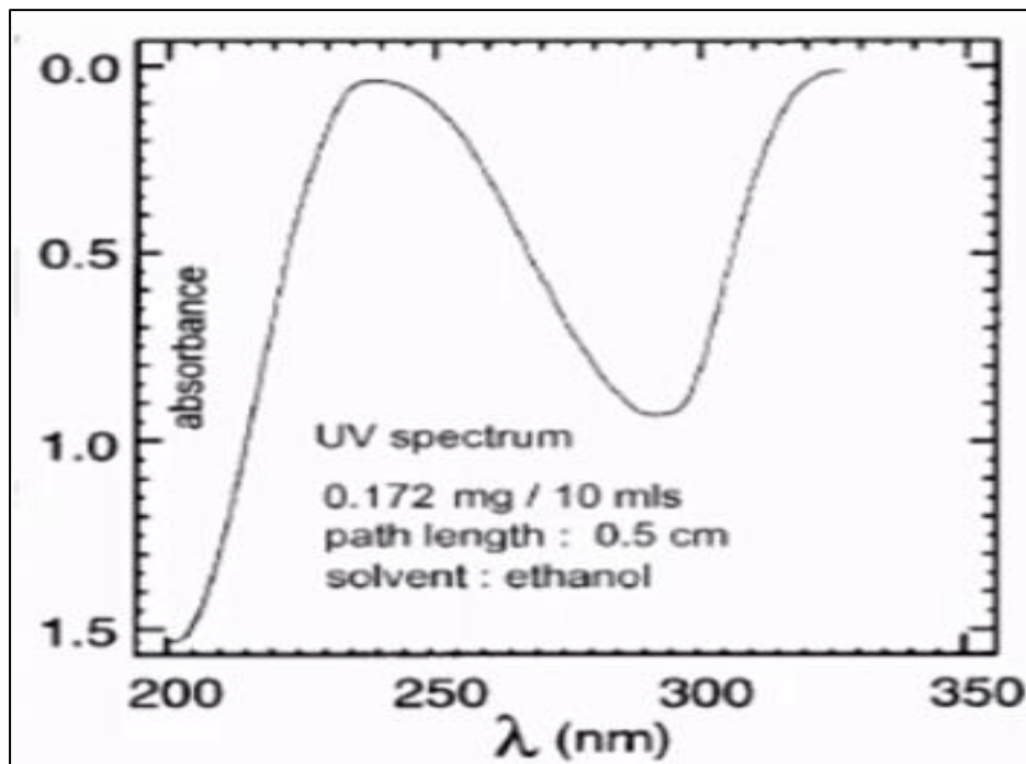
Gambar 2.9 Spektrum UV-Vis menyerupai
