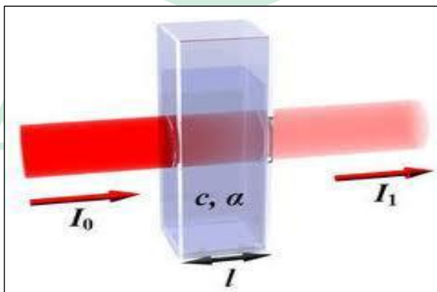
Gambar : 2.8 Proses penyerapan cahaya oleh zat dalam sel sampel.
