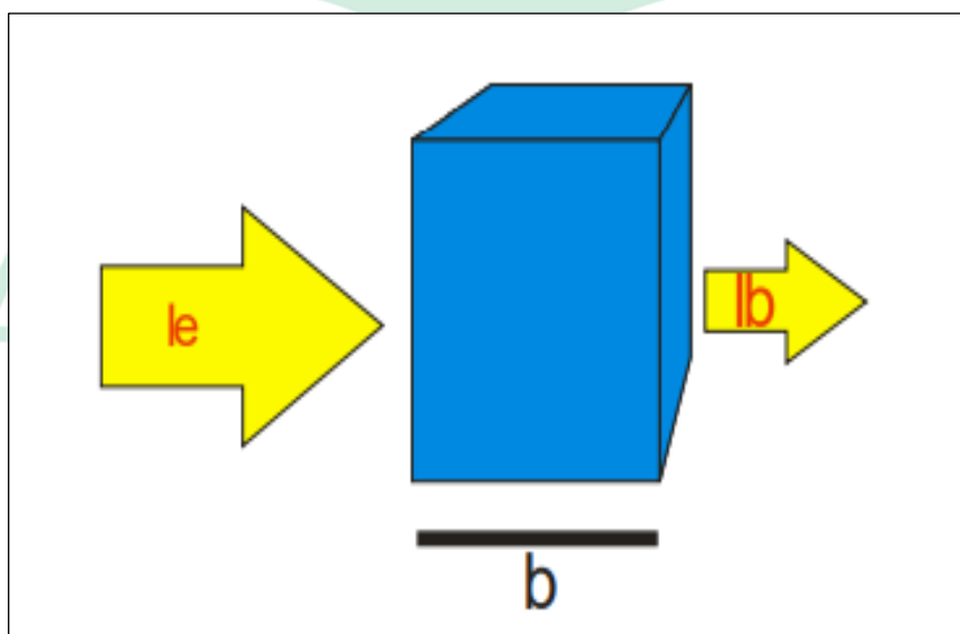
Gambar 2.7: Intensitas cahaya setelah melewati larutan (Sumber: Riski Afandi 2018)
