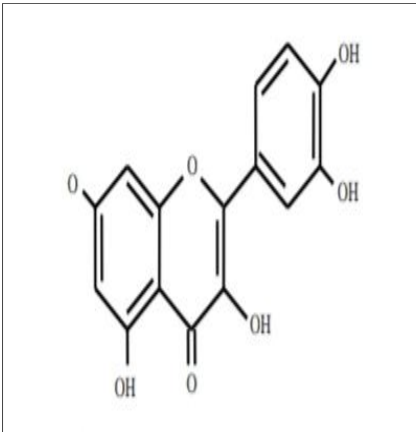
Gambar 2.10 Kerangka C 6 -C 3 -C 6 Flavonoid
