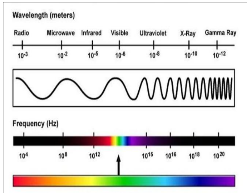
Gambar 2.3 Diagram gelombang elektromagnetik
