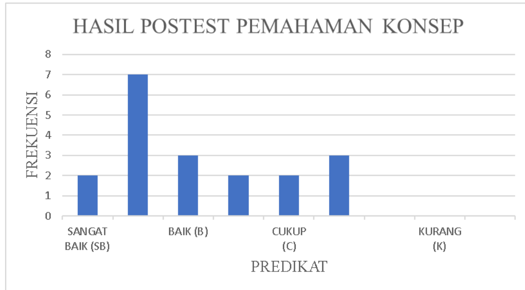
Gambar 4.2 Histogram kategorisasi posttest pemahaman konsep kelas X MIA1
