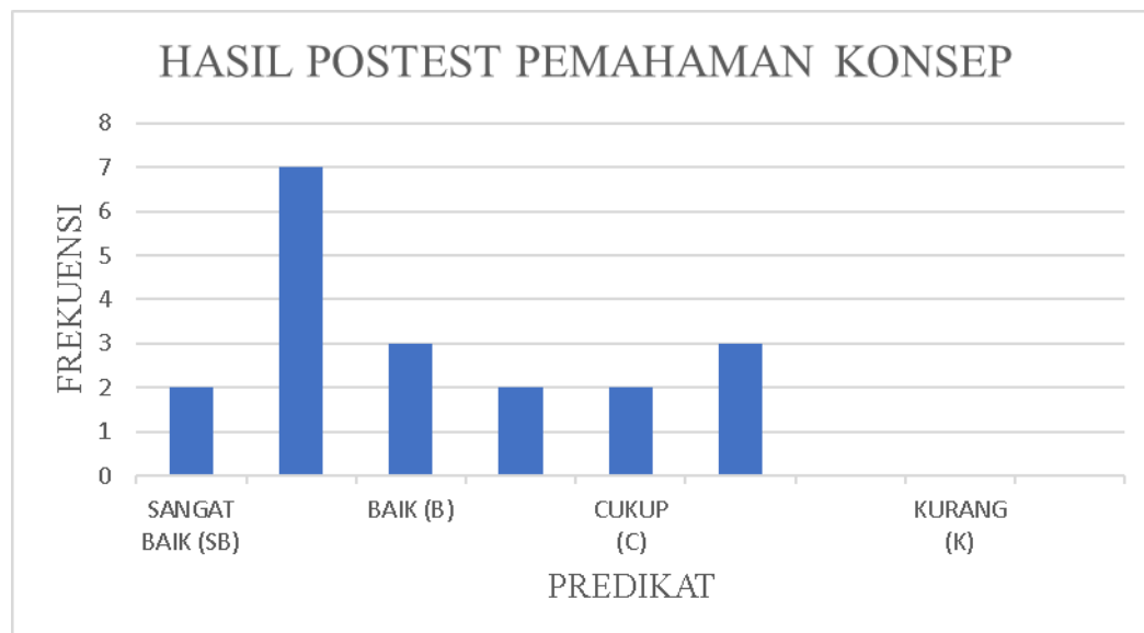
Histogram Posttest Pemahaman Konsep Kelas X MIA 1
