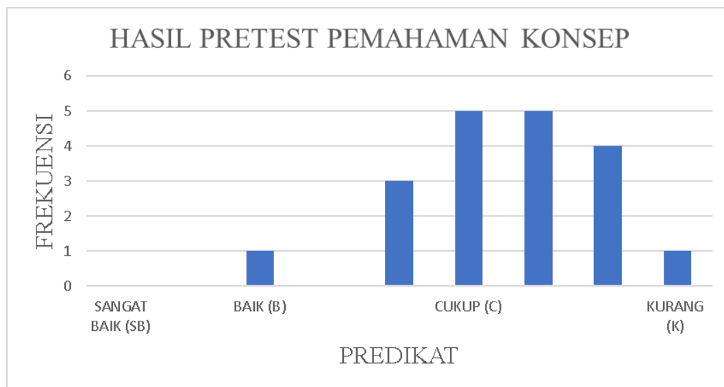
Histogram Pretest Pemahaman Konsep Kelas X MIA 1
