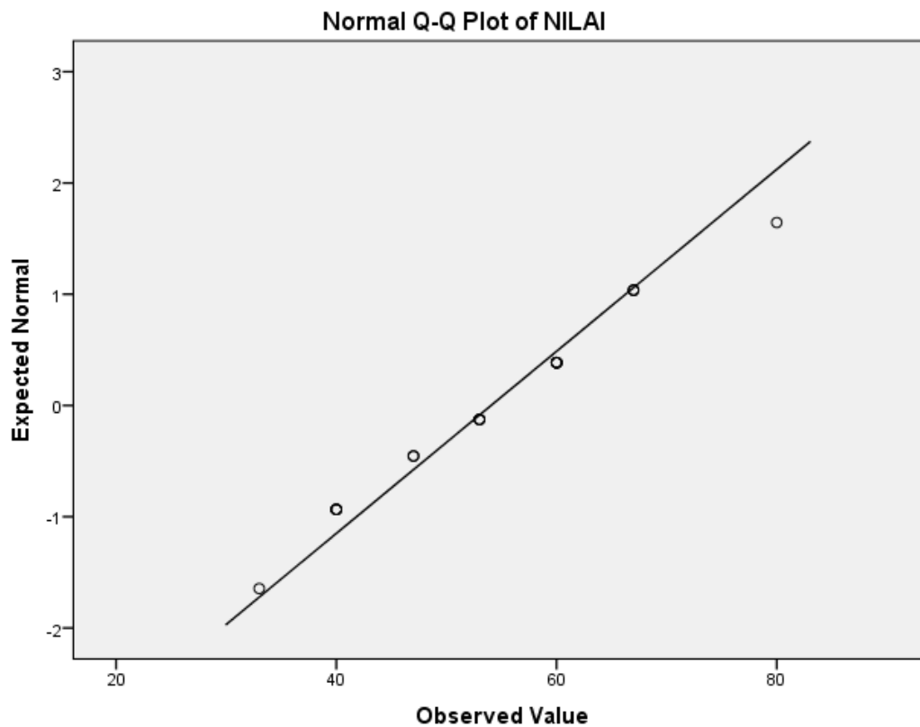
Gambar 4.3 : Grafik Distribusi Normal QQ Plot Pretest Pemahaman Konsep Peserta Didik kelas X MIA 1
