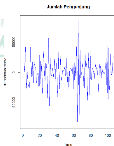
Gambar 4.4 Plot Data Jumlah Pengunjung Wisata Taman Nasional Bantimurung Bulusaraung Maros Setelah Differencing Non Musiman
