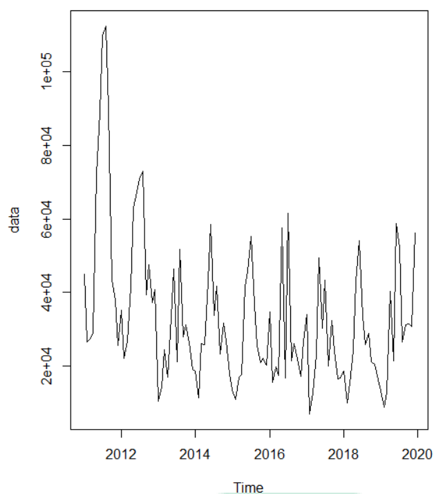
Time Series Plot of Jumlah Pengunjung : 2011-2019
