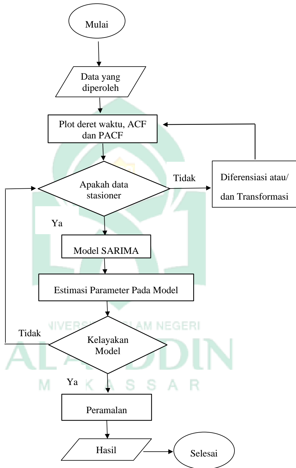
Gambar 3.1 Kerangka Berpikir
