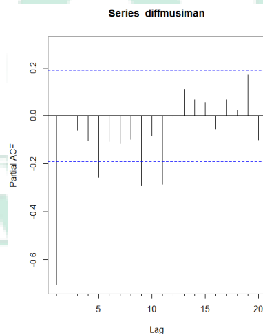
Gambar 4.9 Plot PACF Data Jumlah Pengunjung Wisata Taman Nasional Bantimurung Bulusaraung Maros Setelah Differencing Musiman
