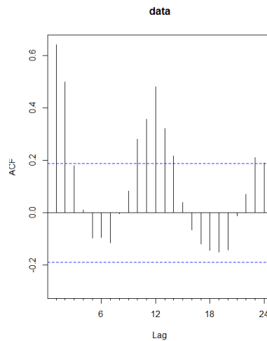
Gambar 4.2 Plot ACF Data Jumlah Pengunjung Wisata Taman Nasional Bantimurung Bulusaraung Maros
