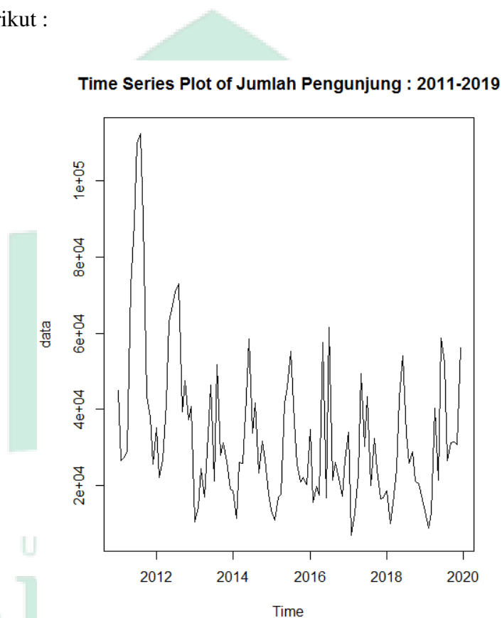
Gambar 4.1 Plot Data Jumlah Pengunjung Wisata Taman Nasional Bantimurung Bulusaraung Maros
