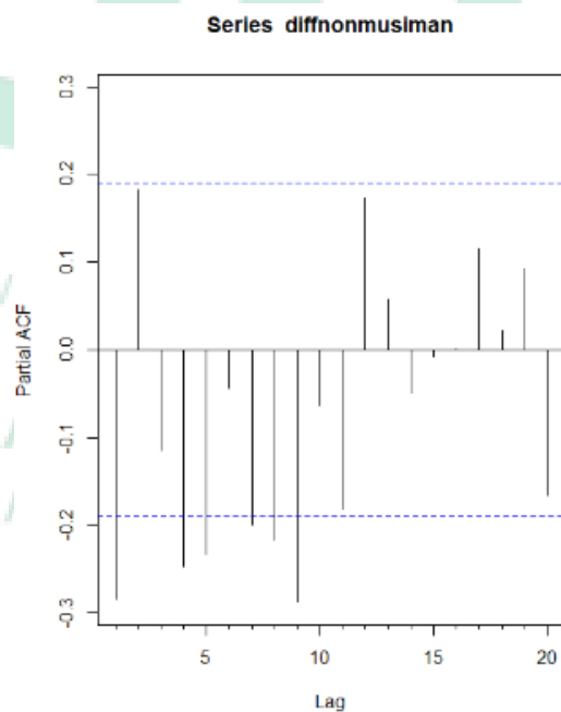
Gambar 4.6 Plot PACF Data Jumlah Pengunjung Wisata Taman Nasional Bantimurung Bulusaraung Maros Setelah Differencing Non Musiman
