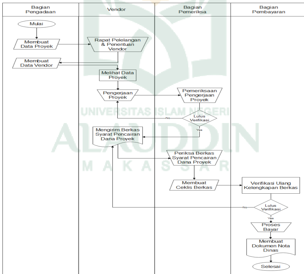
Gambar IV. 1 Flowmap Sistem Yang Sedang Berjalan
