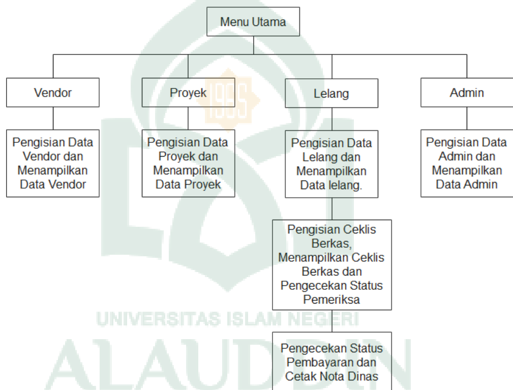
Gambar IV. 13 Struktur Navigasi Administrator
