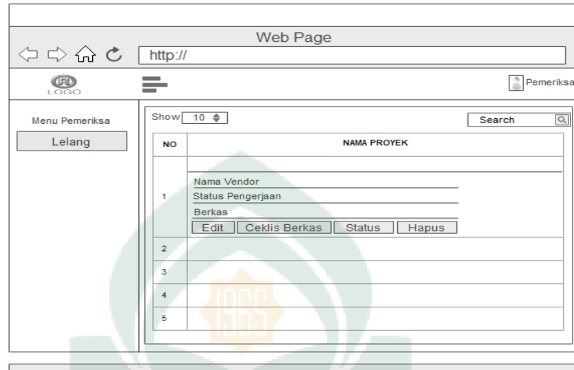
Gambar IV. 21 Tampilan Halaman Lelang
