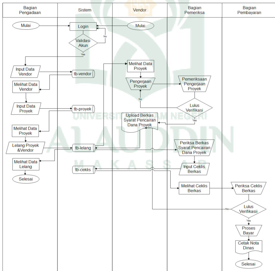
Gambar IV. 2 Flowmap Sistem Yang Diusulkan
