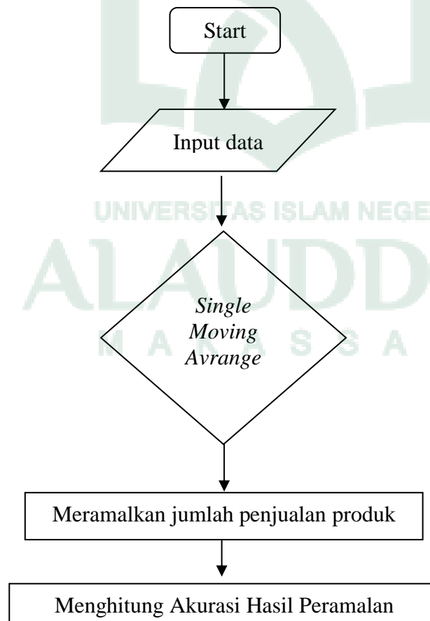
Flowcart Peramalan Menggunakan Single Moving Avarange
