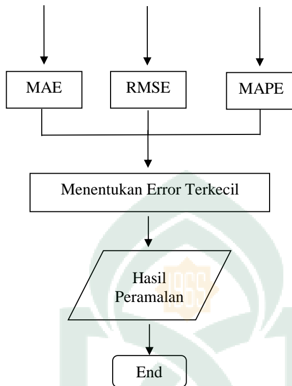
Flowcart Peramalan Menggunakan Single Smooting Eksponensial
