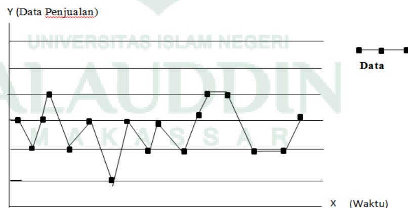
Gambar. 2.6. Single Eksponensial Smooting Pola Horizontal
