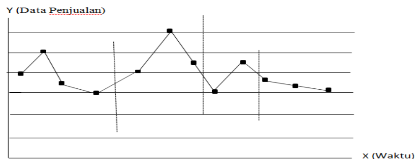
Gambar. 2.8. Triple Eksponensial Smoothing Pola Musiman
