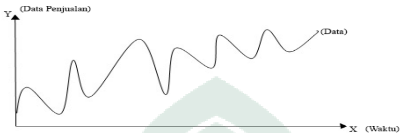
Gambar. 2.4 Variasi Tak Beraturan
