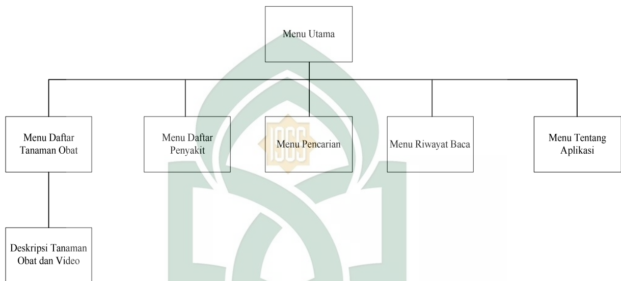
Gambar IV. 10. Struktur Navigasi
