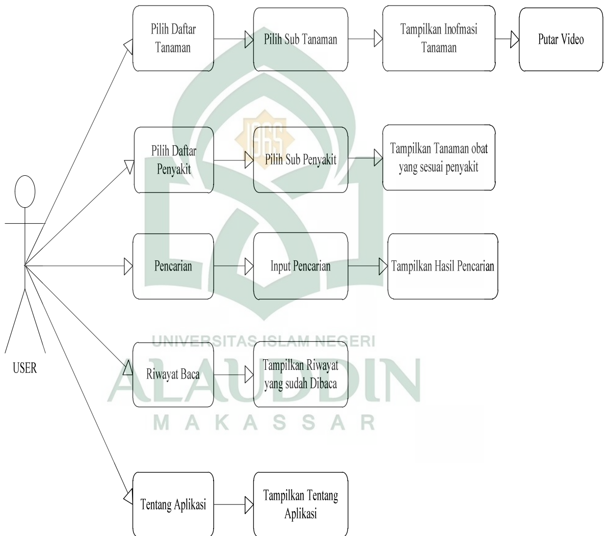
Gambar IV.3. Use Case Diagram Pengguna
