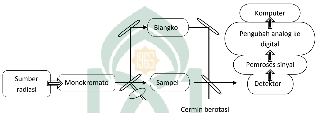
Gambar 2. Skema kerja spektrofotometer UV-Vis (Mulja, 1995).
