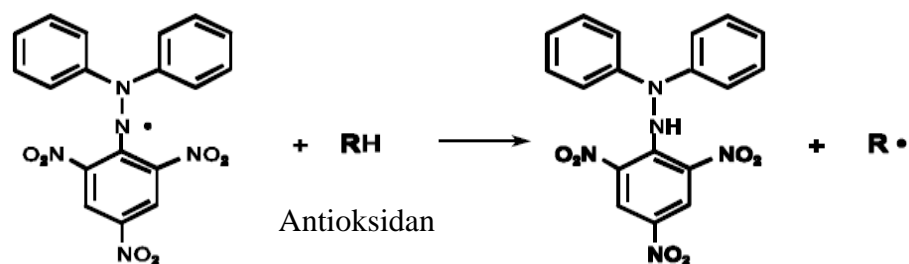
1,1-difenil-2-pikrilhidrazil
