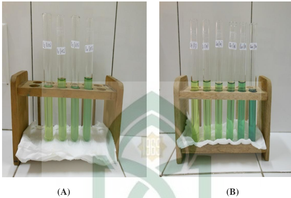
Gambar 13. (A) Sampel buah pare dan (B) Standar kuersetin pada Uji Daya Reduksi Sampel Setelah Penambahan \text{FeCl}_3
