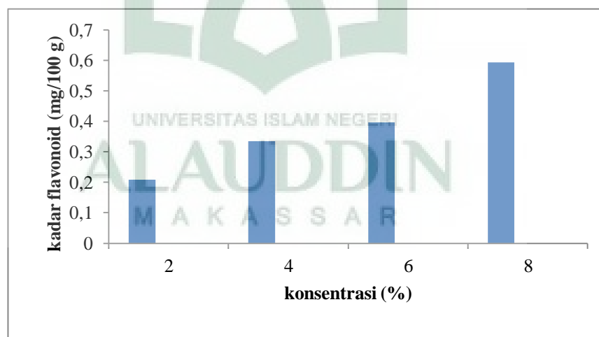
Gambar 5. Grafik Kadar Flavonoid Total pada ekstrak etanol buah pare ( Momordica charantia L)
