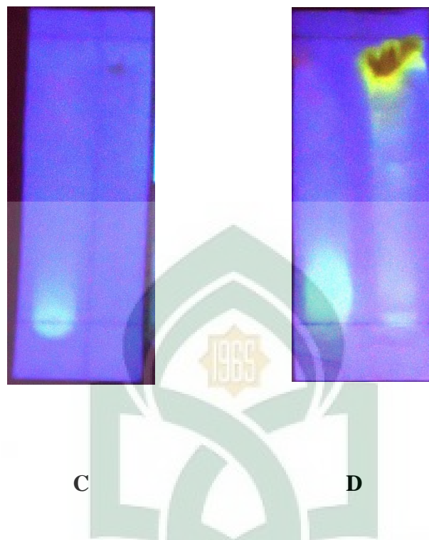
Gambar 10. Foto Profil kromatogram flavonoid sampel buah pare ( Momordica charantia L)
