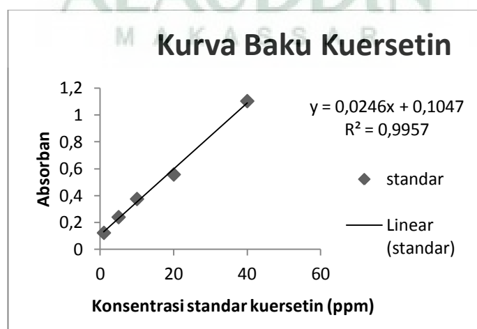
Gambar 4. Grafik perbandingan konsentrasi standar dengan nilai serapannya
