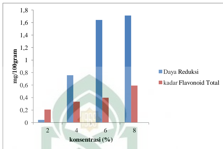
Gambar 8. Hubungan antara kadar flavonoid total dengan daya reduksi pada ekstrak etanol buah pare ( Momordica charantia L)
