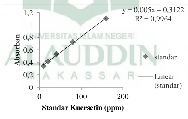
Gambar 6. Grafik perbandingan konsentrasi standar dengan nilai serapannya
