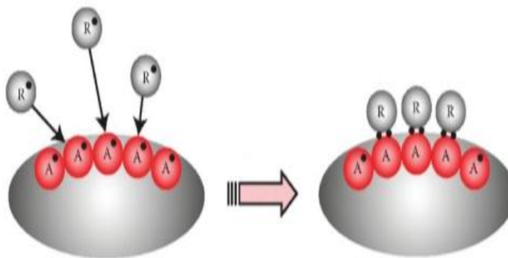
Gambar 4. Ilustrasi Antioksidan ( A^\circ ) dalam Nanopartikel yang Menarik Radikal Bebas ( R^\circ ) ( R:A merupakan senyawa netral) (Mendelson, 2013: 422).
