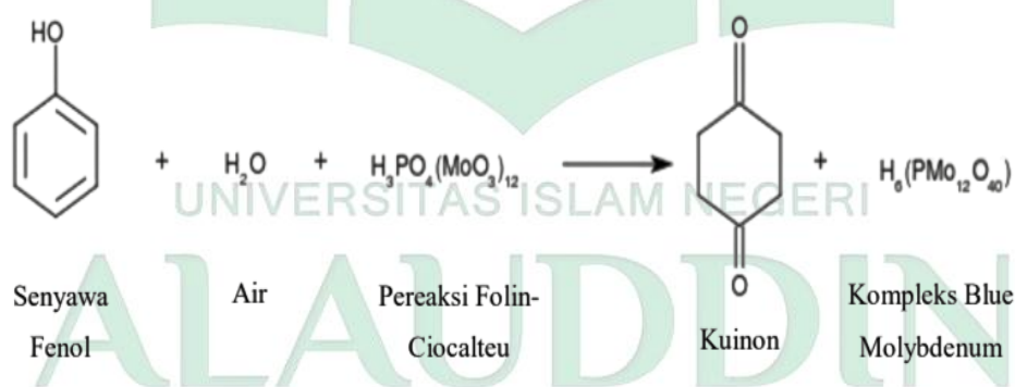
Gambar 6. Reaksi Senyawa Fenolik dengan Reagen Folin-Ciocalteu (Noviyanty et al., 2020: 63).
