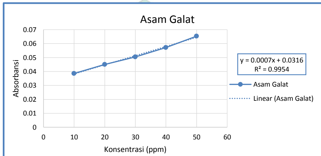
Gambar 9. Kurva Standar Asam Galat
