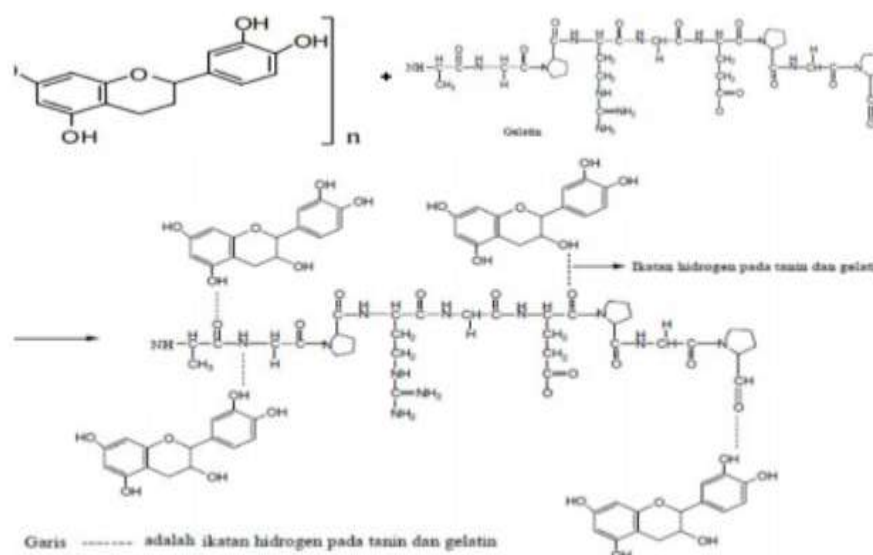
Gambar 6. Reaksi senyawa tanin dan gelatin
