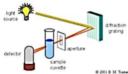
Gambar 7. Skema kerja Spektrofotometri UV-VIS
