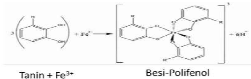
Gambar 5. Reaksi senyawa tanin dengan \text{FeCl}_3
