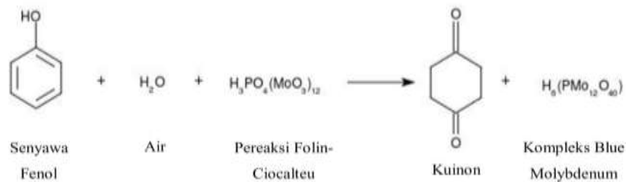
Gambar 7. Reaksi senyawa fenol dengan folin ciocalteu
