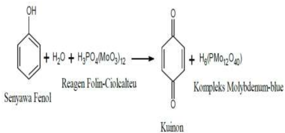
Gambar 6. Reaksi folin ciocalteu dengan fenol
