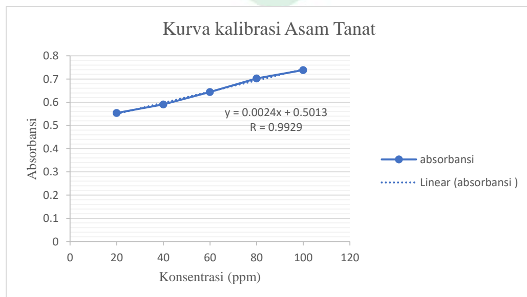
Gambar 8. Kurva baku asam tanat
