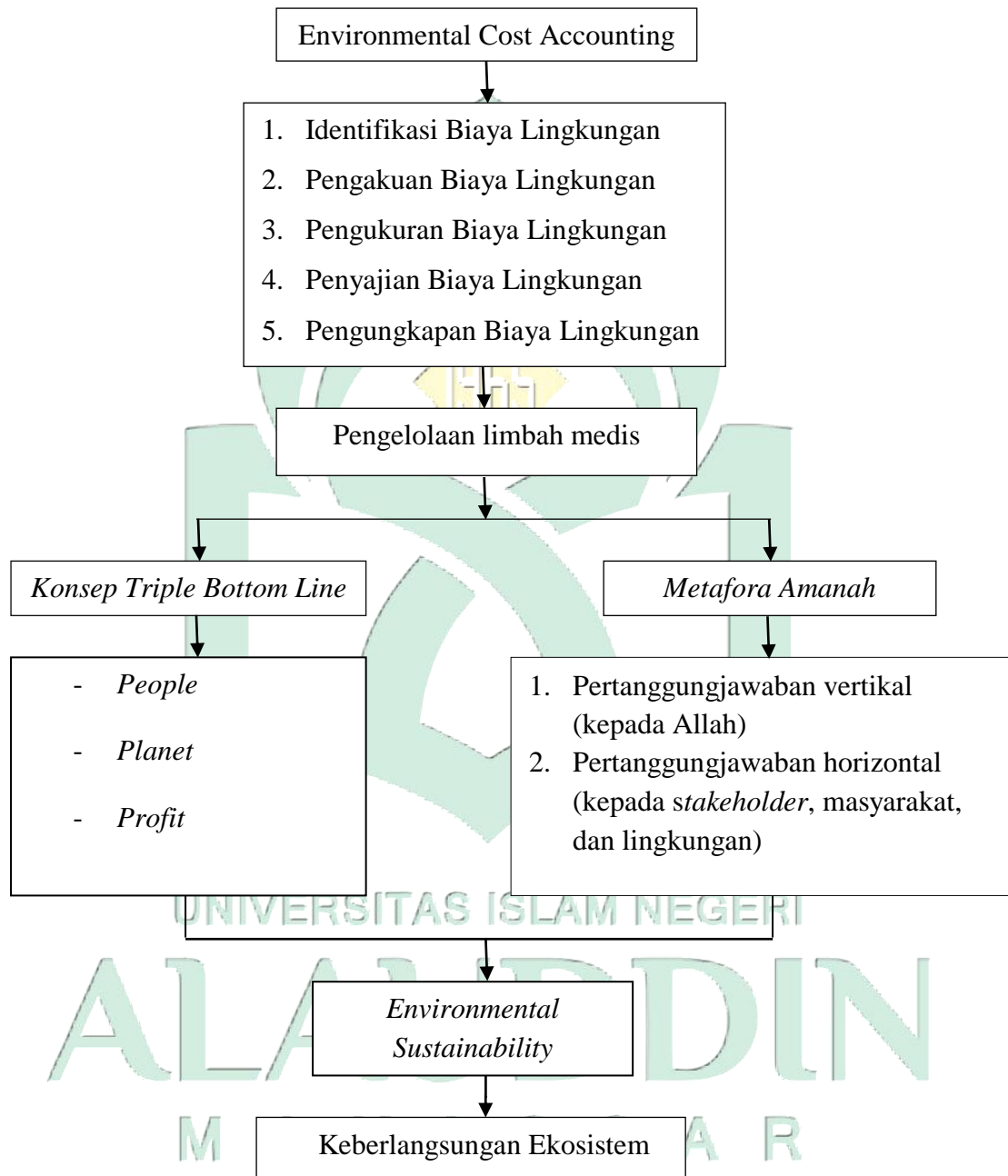
Gambar 2.1 Rerangka Pikir
