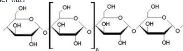
Gambar 5. Struktur pati
