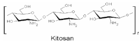
Gambar 3. Struktur kitosan
