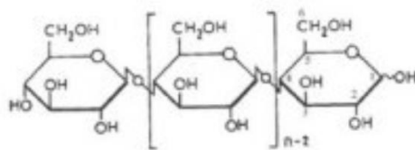
Gambar 4. Struktur selulosa
