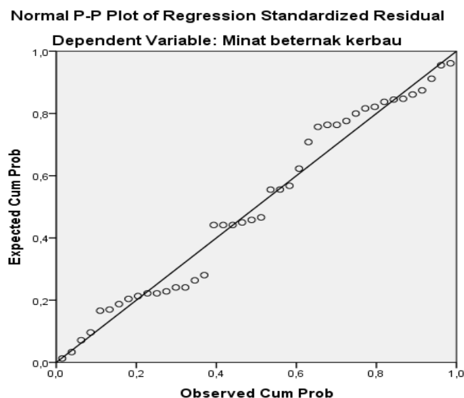
Gambar 3. Diagram penyebaran nilai variabel independent terhadap variabel dependen.
