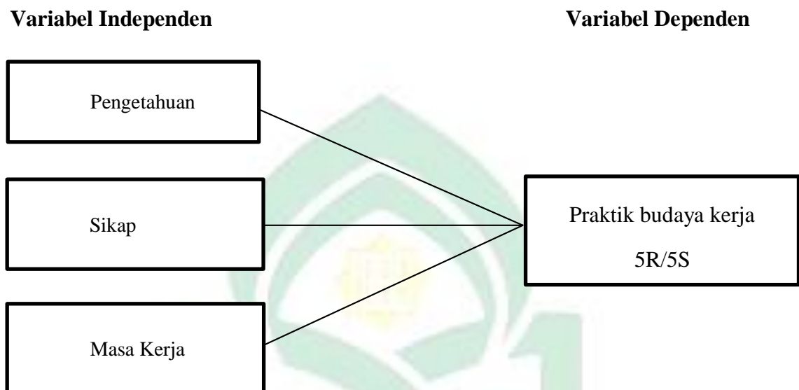
Gambar 2.6 Kerangka Konsep
