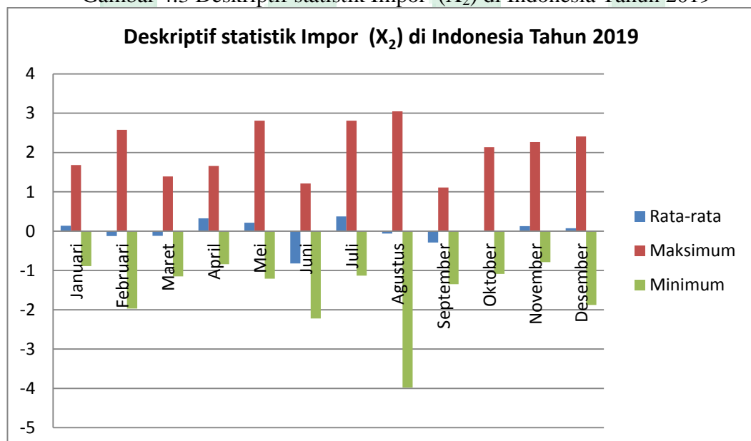
Gambar 4.3 Deskriptif statistik Impor ( X_2 ) di Indonesia Tahun 2019
