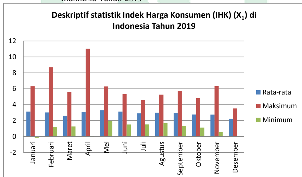
Gambar 4.2 Deskriptif statistik Indeks Harga Konsumen (IHK) ( X_1 ) di Indonesia Tahun 2019
