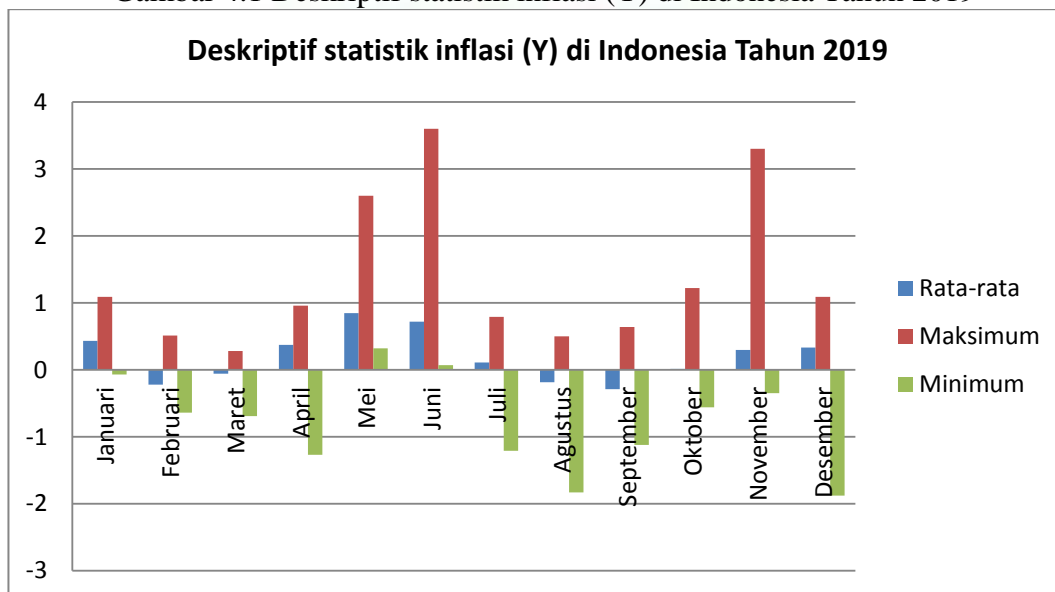
Gambar 4.1 Deskriptif statistik inflasi (Y) di Indonesia Tahun 2019
