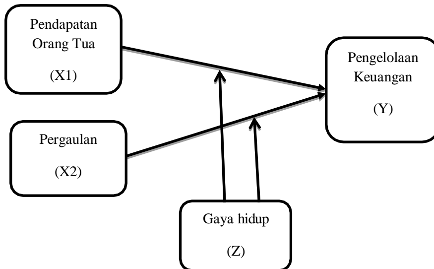
Gambar 2.1 Kerangka Pikir
