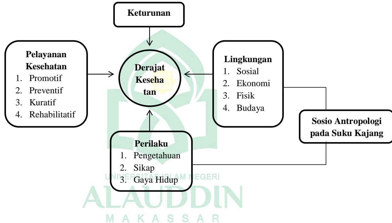
Gambar 2.1 Kerangka Teori
