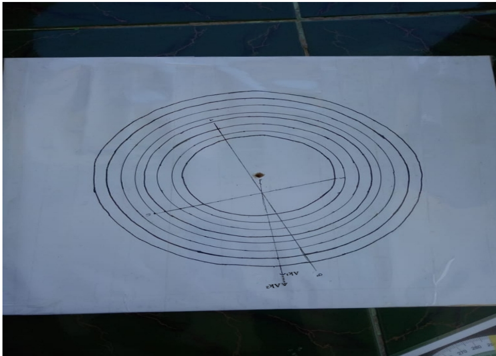
Gambar. 3 Hasil Pengukuran Arah Kiblat dengan Menggunakan Tongkat Istiwa'
