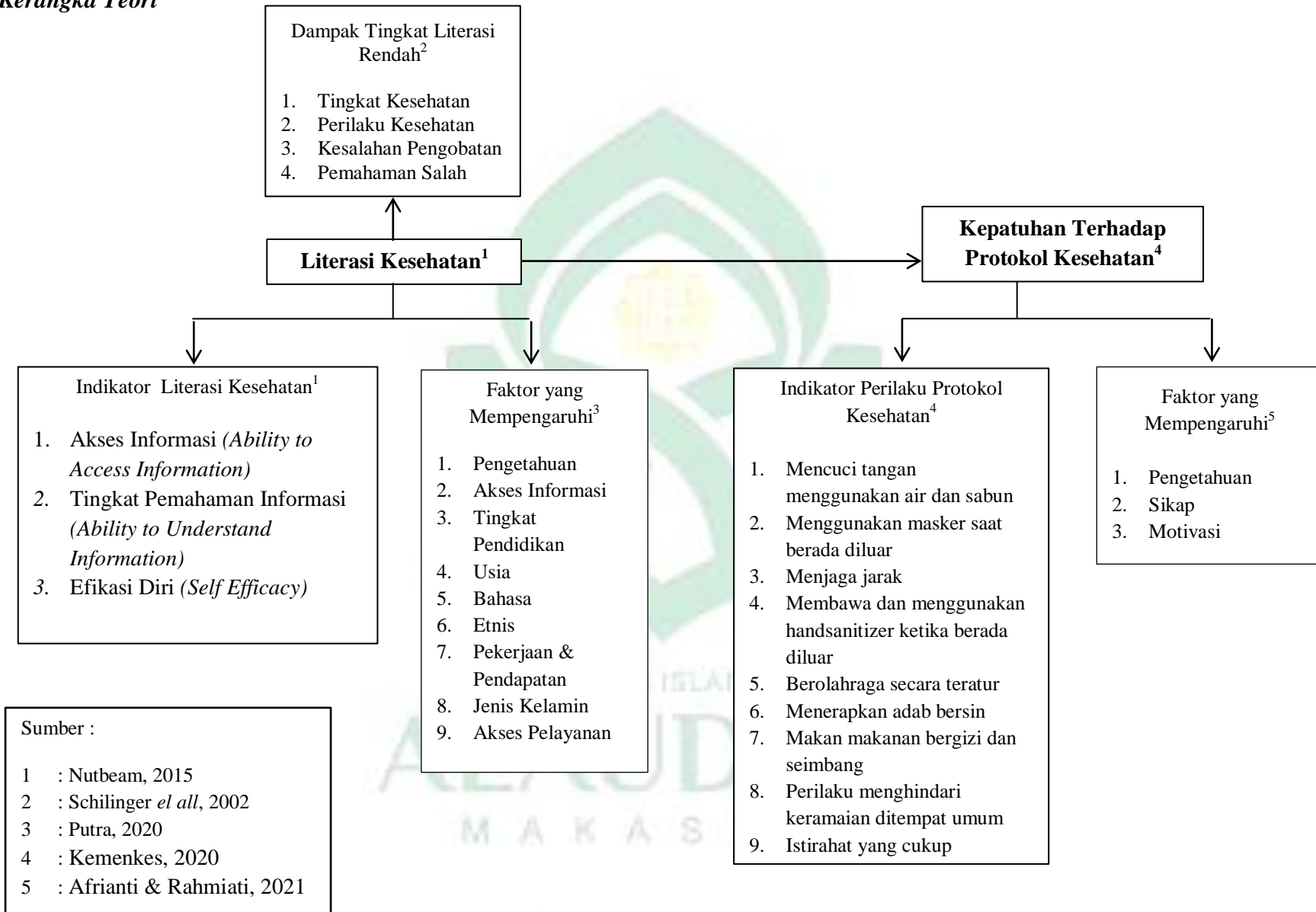
Gambar 2.3 Kerangka Teori
