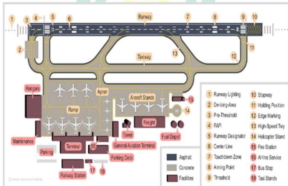
Gambar II.1 Contoh infrastruktur Bandar udara Sumber : http://astrophysicsblogspot.com , (diakses 15 september 2019)
