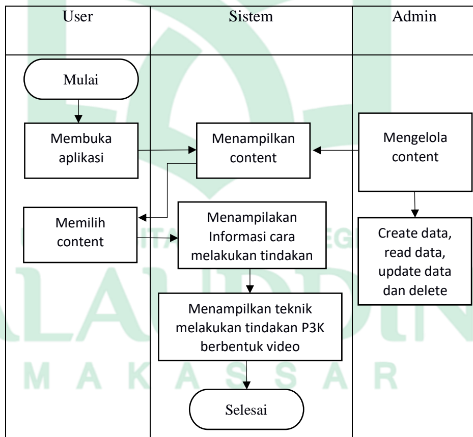
Gambar IV.2. Flowmap sistem yang diusulkan
