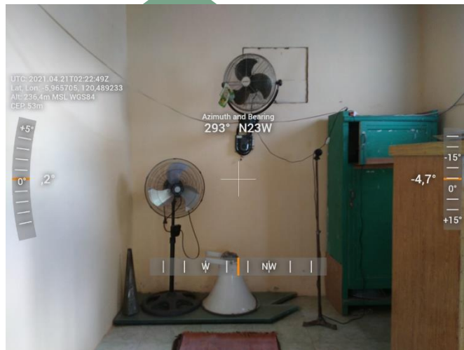
Gambar 1.8 Pengukuran Arah Kiblat Masjid Nurul Amin Dusun Toge' Desa Kayu Bauk Kecamatan Bontomatene Kabupaten Selayar menggunakan Dioptra.
