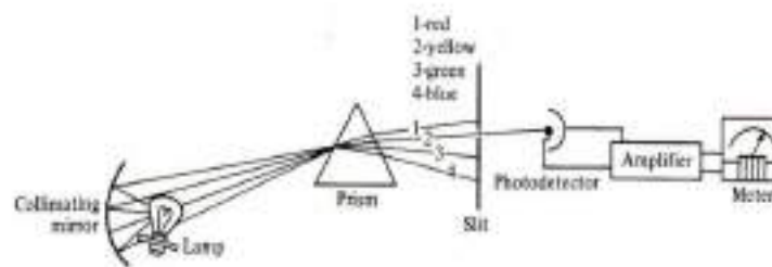
Gambar 4. Skema spektrofotometer Uv-Vis
