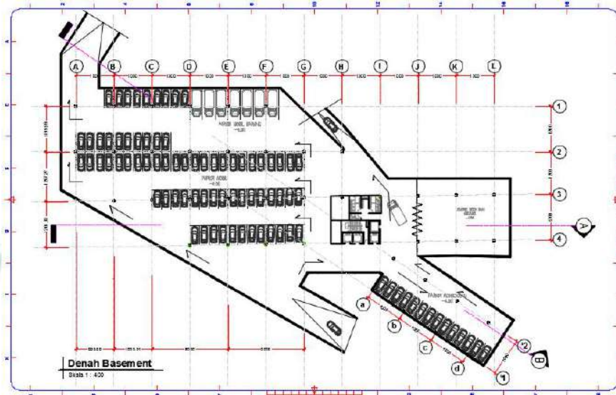
Gambar VI.2 Denah lantai basement Sumber : Olah desain, 2020
