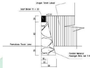
Gambar III.9 Pondasi batu kali
