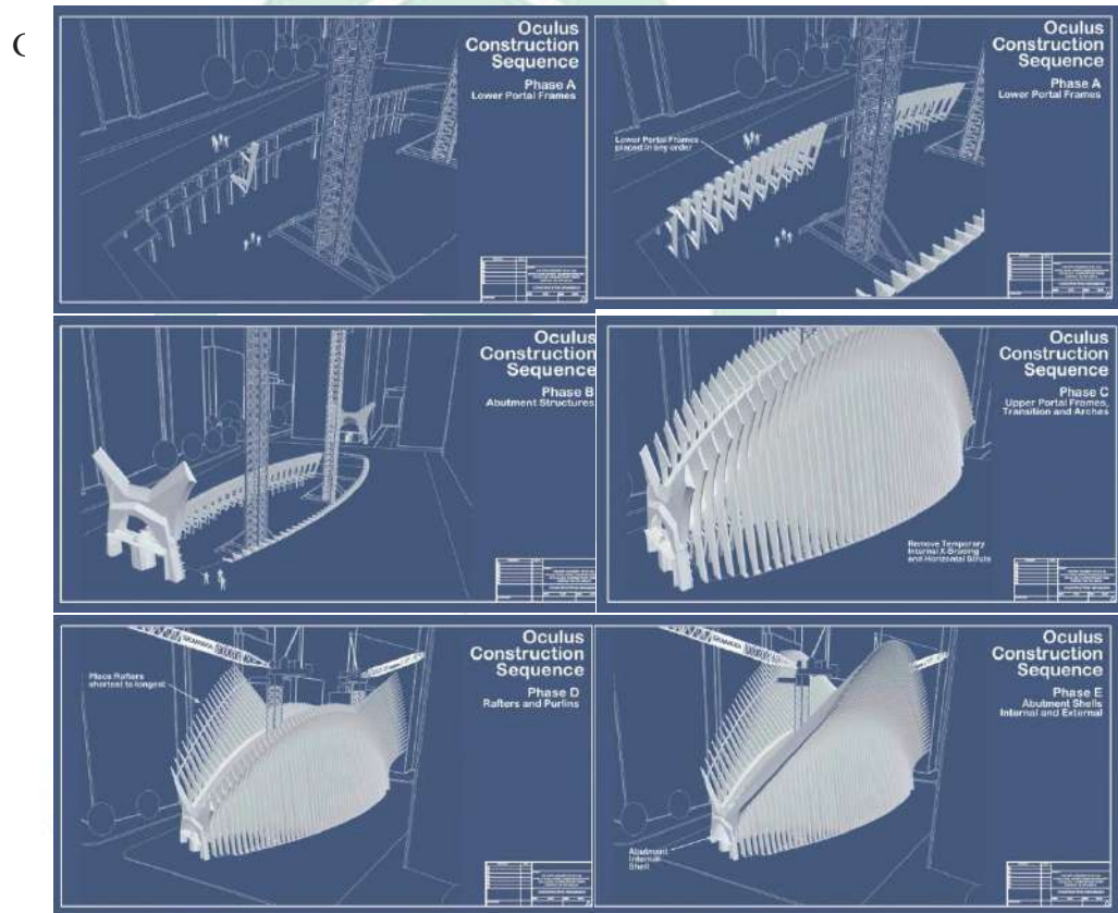
asangan Struktur Rangka Oculus Sumber: archdaily.com
