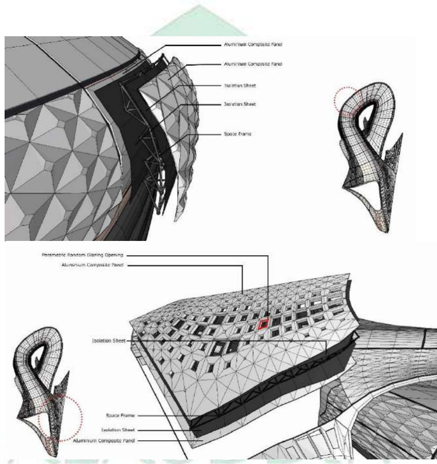
Gambar VI.12 Detail Struktur dan konstruksi Sumber : Olah desain, 2020
