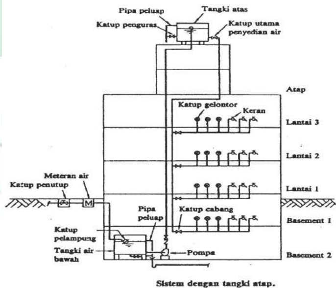
Gambar III.3 Sistem tangki atap Sumber : lingkunganitats.wordpress.com , diakses september 2019
