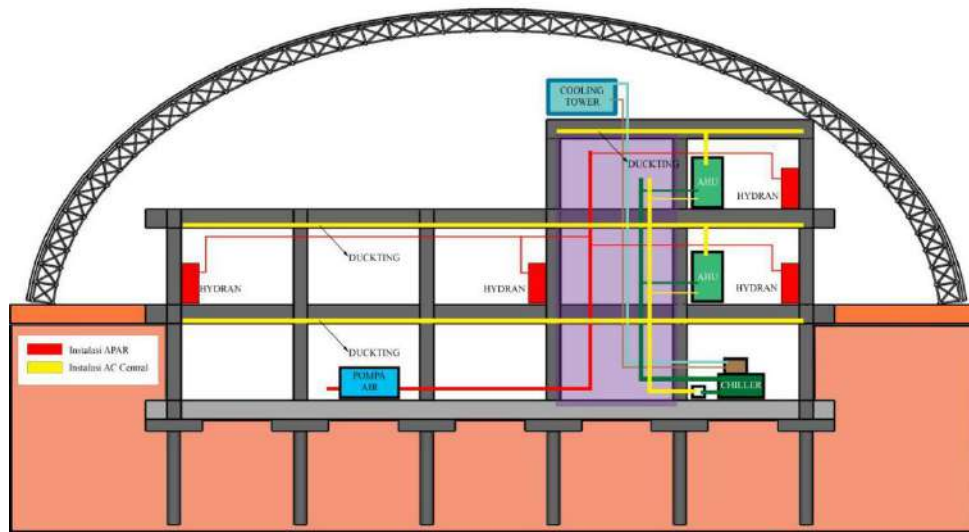
Gambar IV.38 Ilustrasi Sistem Penyejuk ruangan, Sistem APAR Sumber : Olah data Lapangan, 2019
