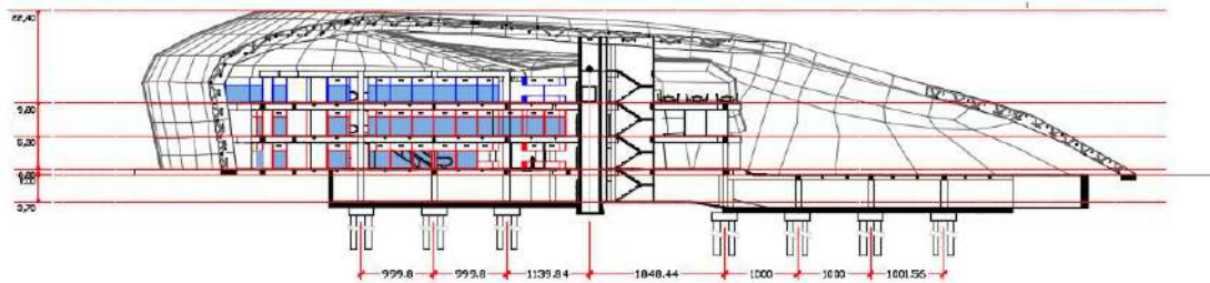
Potongan A-A Skala 1 : 500
