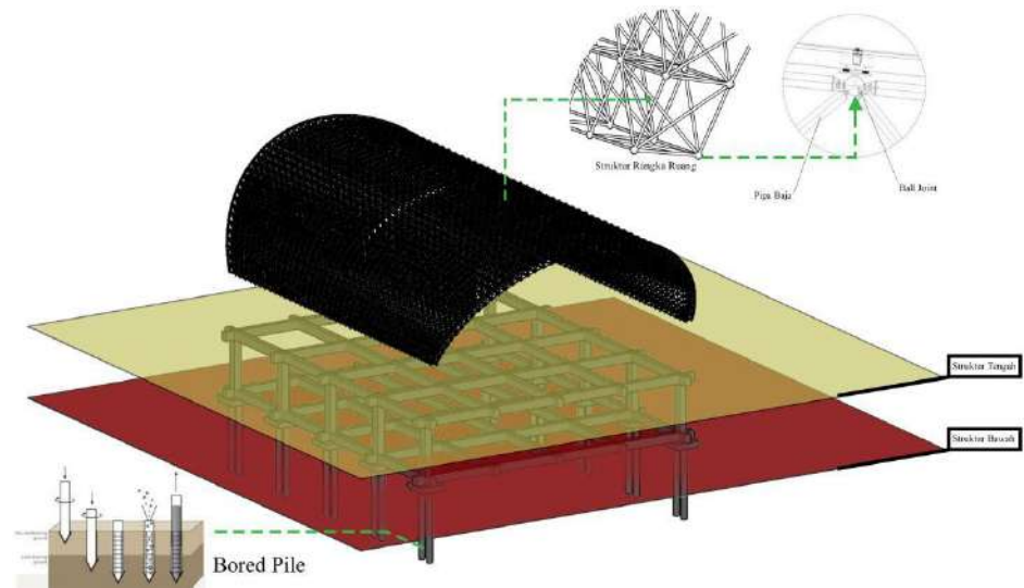
Gambar IV.37 Konsep Struktur Bangunan Sumber : Olah data Lapangan, 2019
