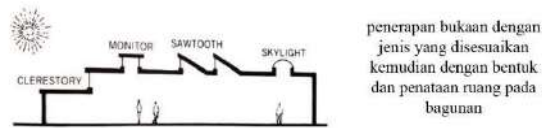
Gambar IV.19 Tanggapan Terhadap Matahari Sumber : Olah Data, 2019
