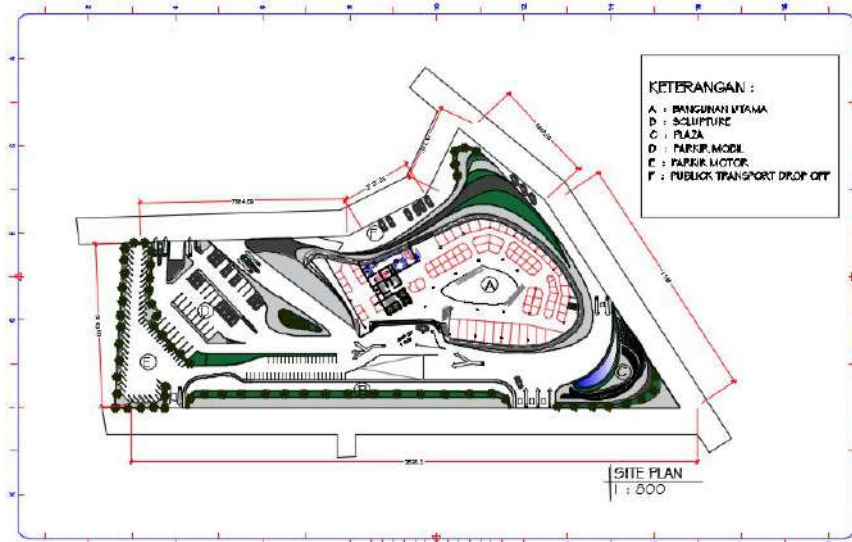
Gambar VI.1 Site Plan Sumber : Olah desain, 2020
