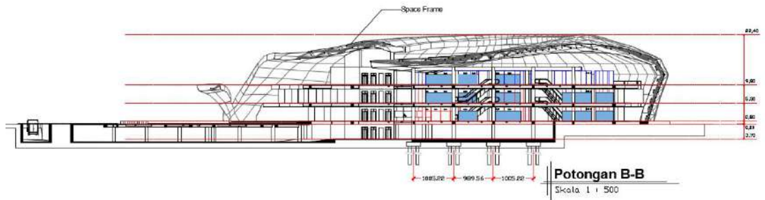
Gambar VI.11 Potongan B-B Sumber : Olah desain, 2020
