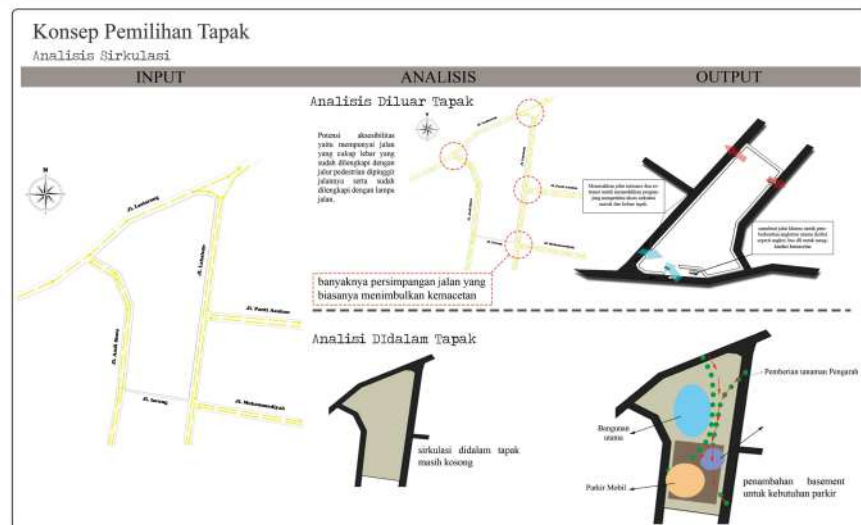
Gambar V.3 Analisis akhir pengolahan tapak (sirkulasi) Sumber : Olah desain, 2020
