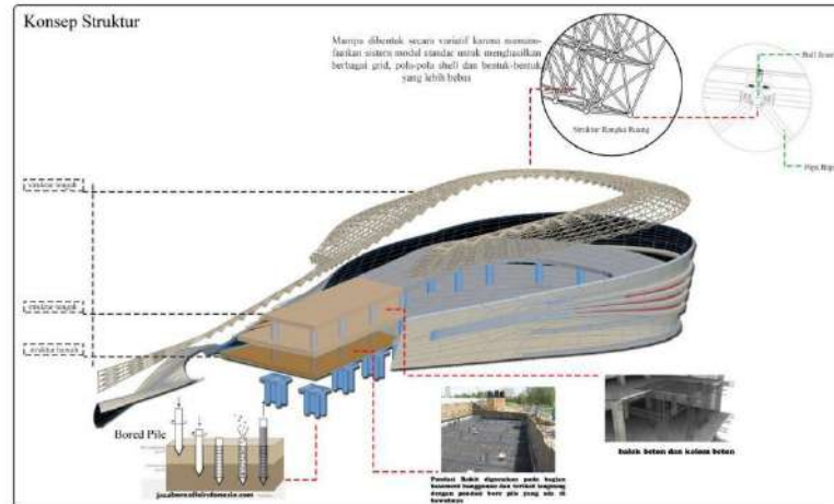
Gambar V.14 Analisis struktur bangunan Sumber : Olah desain, 2020
