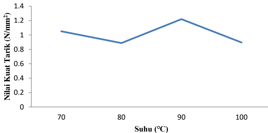
Gambar 4.4 Hubungan Variasi Suhu dengan Kuat Tarik
