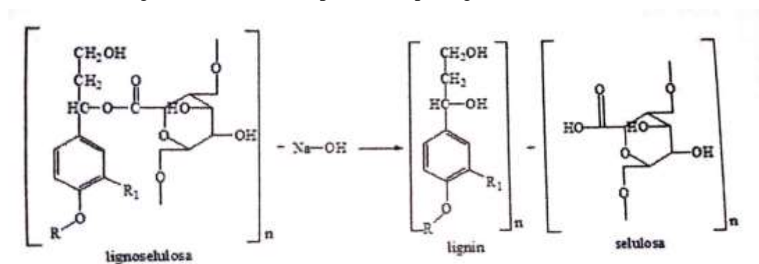
Gambar 4.3 Reaksi proses delignifikasi (Sumber: Rahmidar, dkk., 2018)
