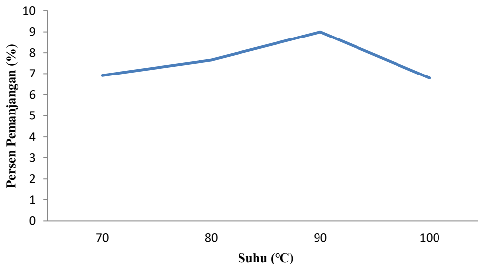
Gambar 4.5 Hubungan Variasi Suhu dengan Nilai Persen Pemanjangan
