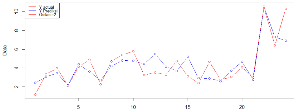
Gambar 4.28 Perbandingan estimasi dengan data model 2 titik osilasi
