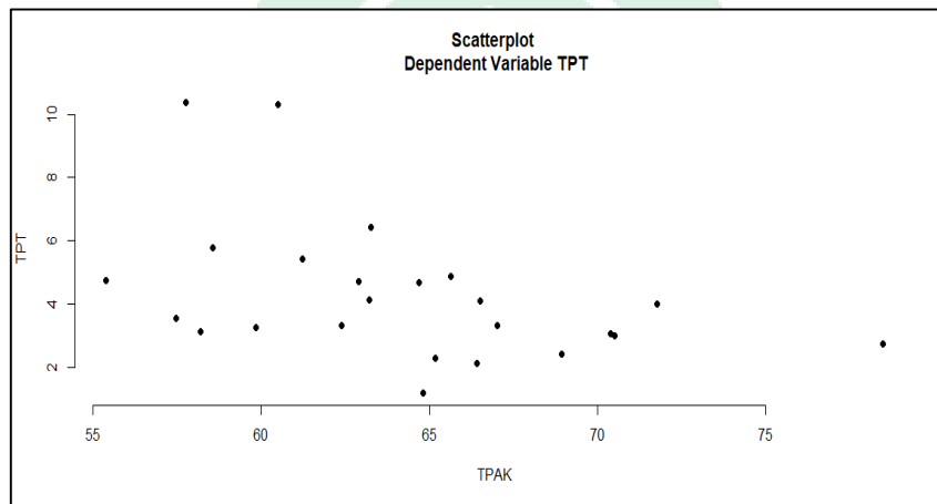
Gambar 4.14 Scatterplot antara TPT ( Y ) dengan TPAK ( X_3 )
