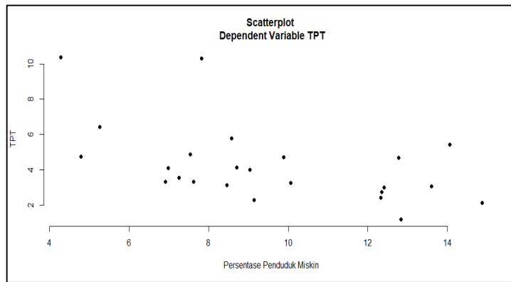
Gambar 4.23 Scatterplot antara TPT ( Y ) dengan Persentase Penduduk Miskin ( X_5 )
