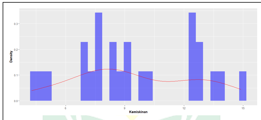
Gambar 4.25 Plot Skewness dan Kurtosis Data Persentase Penduduk Miskin
