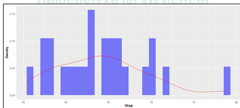
Gambar 4.16 Plot Skewness dan Kurtosis Data Tingkat Partisipasi Angkatan Kerja
