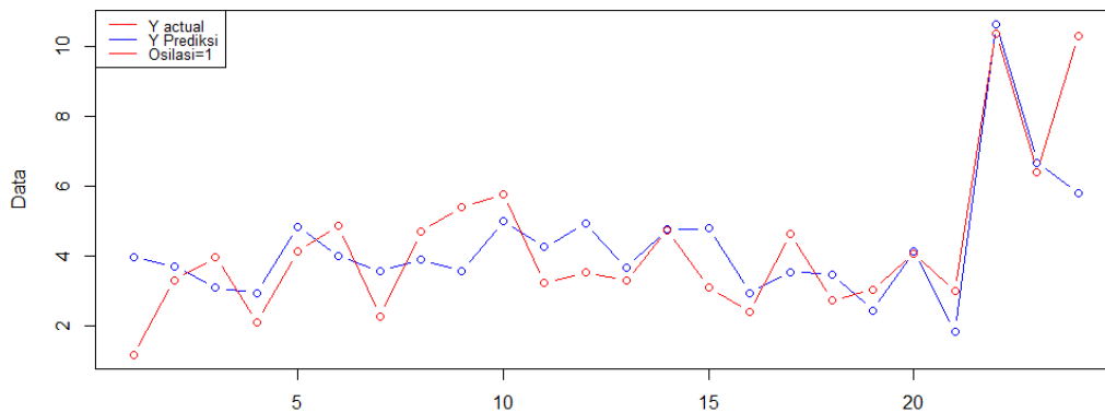
Gambar 4.27 Perbandingan estimasi dengan data model 1 titik osilasi
