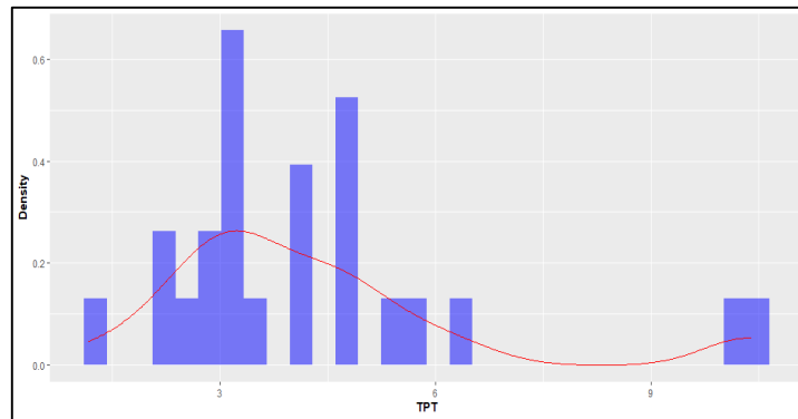
Gambar 4.4 Plot Skewness dan Kurtosis Data Tingkat Pengangguran Terbuka
