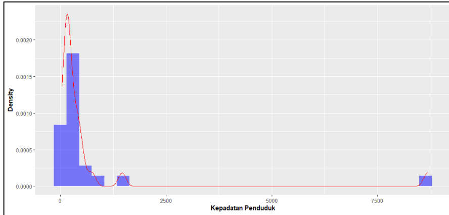
Gambar 4.8 Plot Skewness dan Kurtosis Data Kepadatan Penduduk
