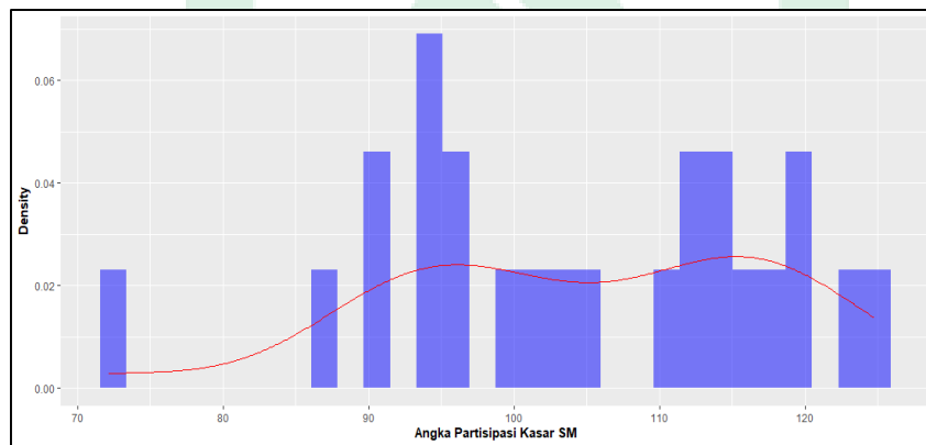
Gambar 4.20 Plot Skewness dan Kurtosis Data Angka Partisipasi Kasar SM
