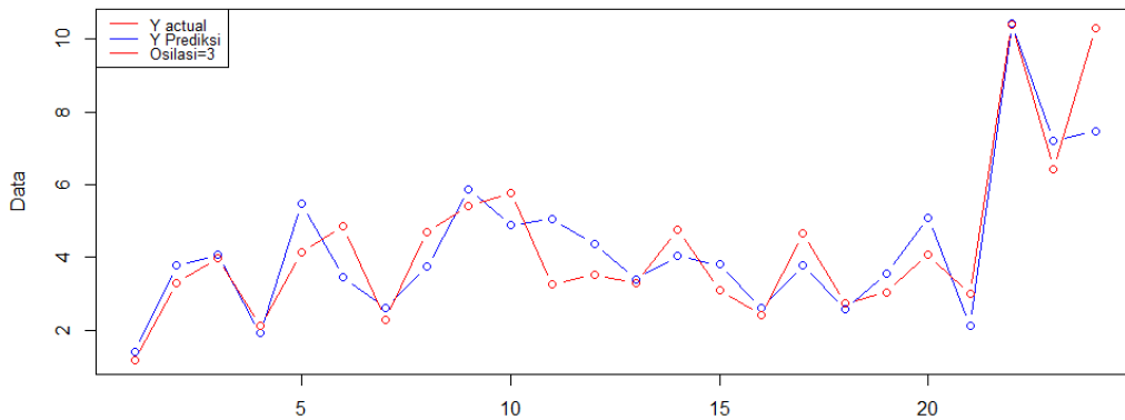
Gambar 4.29 Perbandingan estimasi dengan data model 3 titik osilasi
