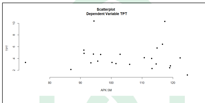
Gambar 4.18 Scatterplot antara TPT (Y) dengan APK SM ( X_4 )
