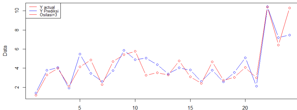
Gambar 4.40 Perbandingan Hasil Prediktor dengan Data Aktual
