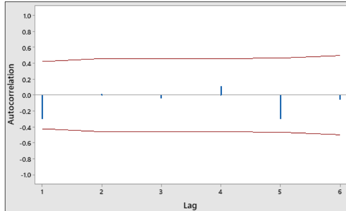
Gambar 4.34 ACF dari Residual
