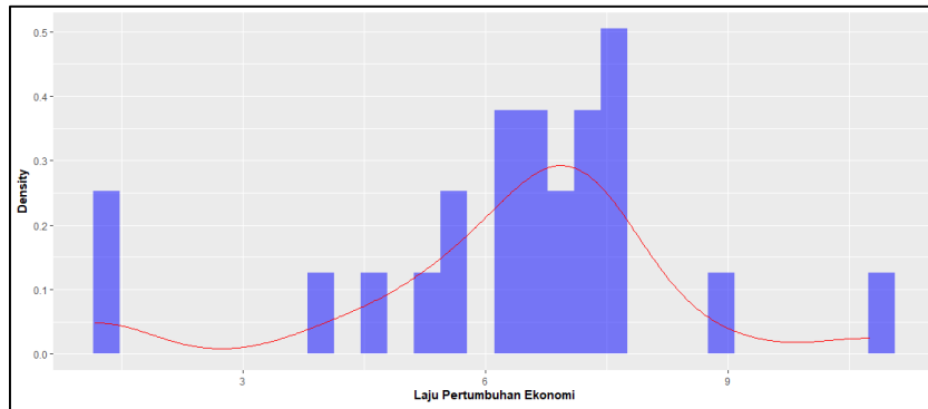
Gambar 4.12 Plot Skewness dan Kurtosis Data Laju Pertumbuhan Ekonomi
